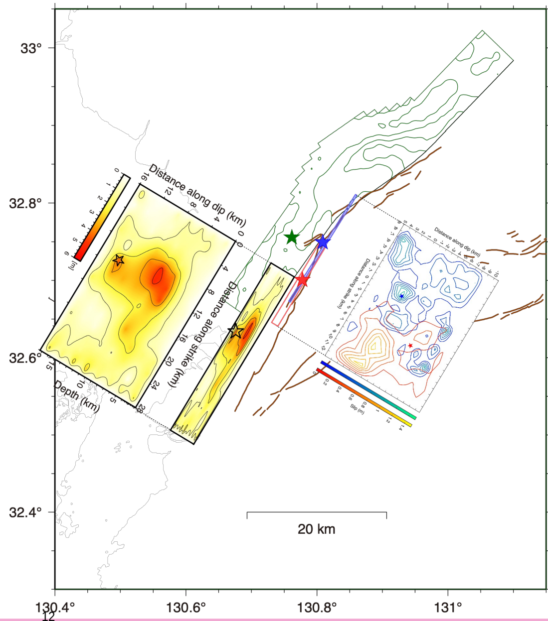
図6：令和8年熊本地震のすべり分布と過去の大規模地震のすべり分布の空間比較。令和8年熊本地震のすべり分布の地表投影をカラーで、破壊開始点を黒星で示す。黒のコンターは1.2m毎のすべり量を示す。2016年4月16日1時25分頃に発生した M_j7.3 の平成28年熊本地震の震央を緑の星で、すべり分布を緑のコンターで示す(Kubo et al., 2016, EPS)。緑のコンターは0.8m毎のすべり量を表す。青の星と矩形は2016年4月14日21時26分頃に発生した M_j6.5 の地震の震央と断層面を表す。赤の星と矩形は2016年4月15日0時3分頃に発生した M_j6.4 の地震の震央と断層面を示す。青と赤のコンターはそれぞれ M_j6.5 の地震と M_j6.4 の地震の0.2m毎の断層すべり分布を表す(Shibata and Aso, 2025, BSSA, 図11に加筆修正)。茶色線はAIST (2007) による活断層の地表トレースを表す。
