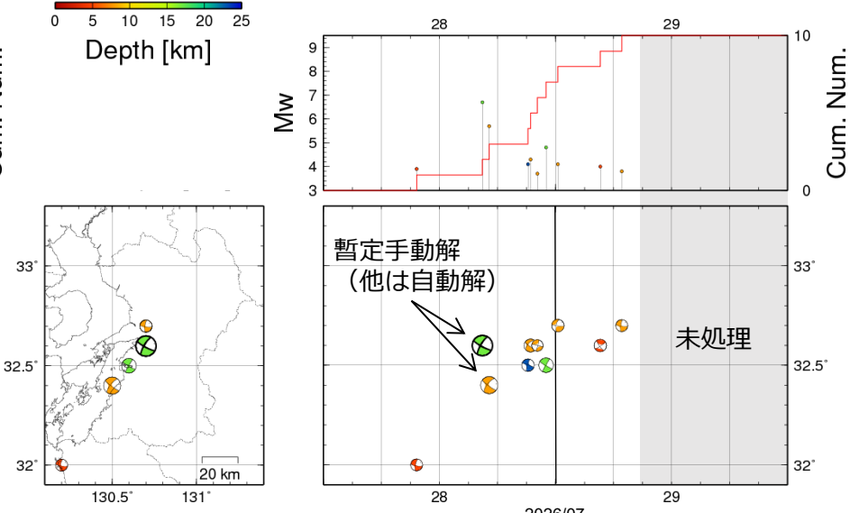
図2 図1のうち2026年7月28日以降の地震.
