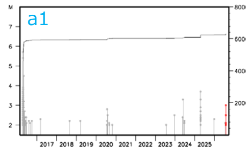
領域a1～a4内のM-T図及び回数積算図
