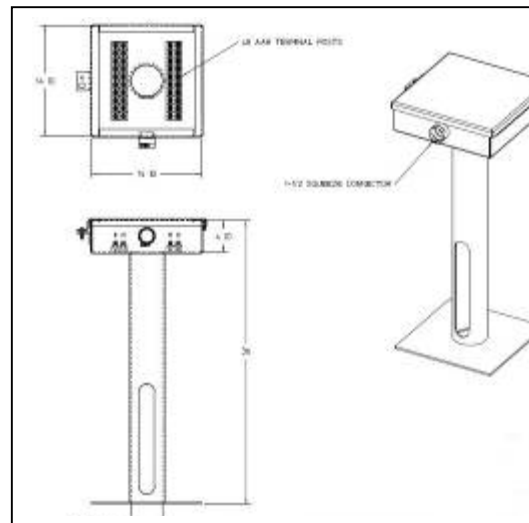
3A7006-021 - 20 WAY
