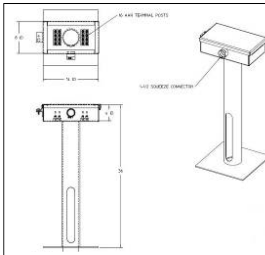
3A7006-011 - 8 WAY
