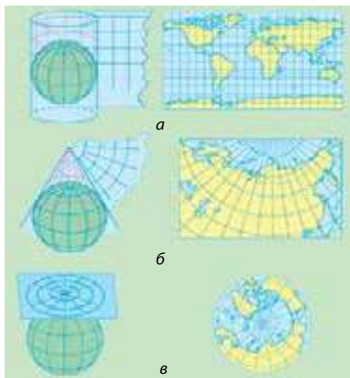
Мал. 34. Картографічні проєкції за видом допоміжної поверхні: а – циліндрична; б – конічна; в – азимутальна
