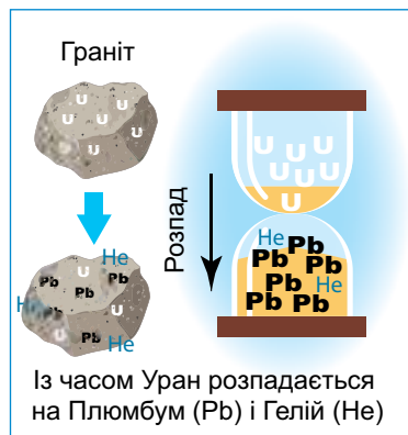
Мал. 53. Радіометричний метод визначення віку порід за часом напіврозпаду радіоактивних елементів
