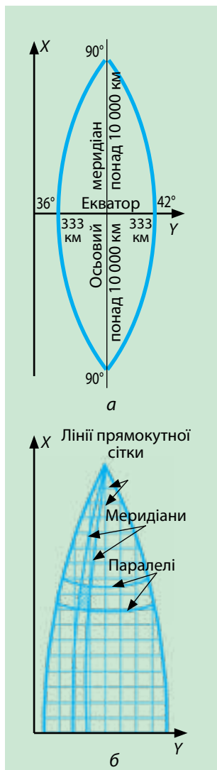
Мал. 42. Зональна система прямокутних координат
