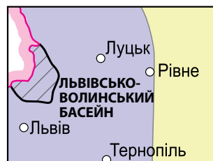
Спосіб ареалів
