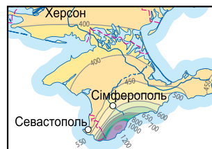
Спосіб ізоліній
