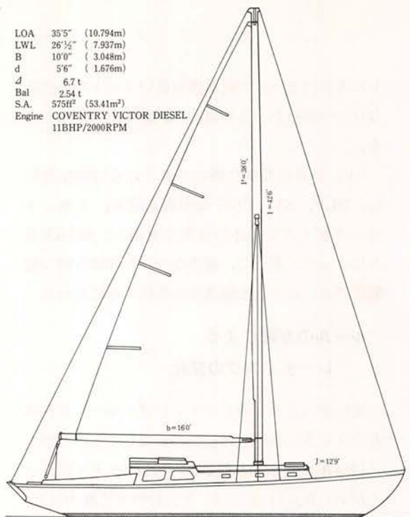
Fig 8 「コンテッサⅡ」のセールプラン
