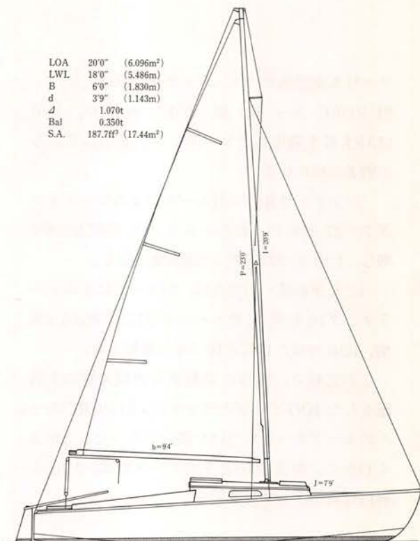
Fig 6 「どんがめIV」のセールプラン
