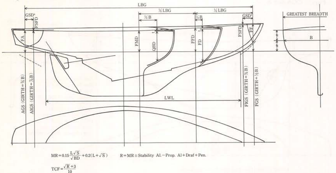
Fig 3 RORC ルール（1957年）
