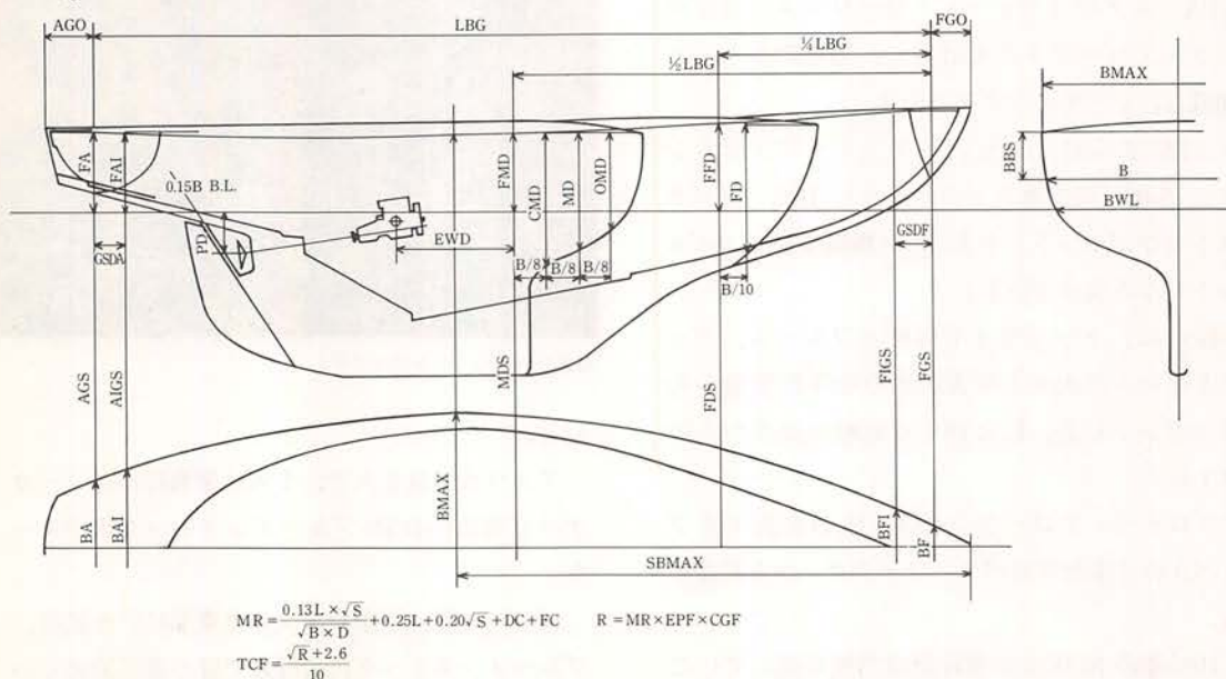
Fig 4 IOR ルール MARK II
