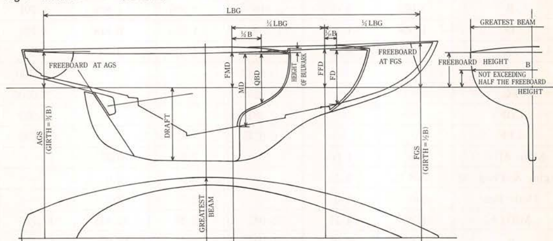
Fig 1 RORCルール(1949年)
