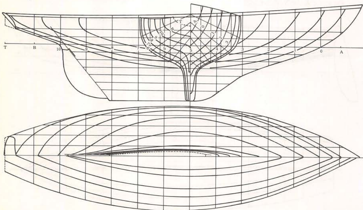
Fig 7 「コンテッサⅡ」のライン図
