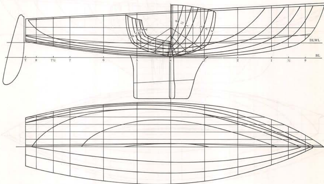
Fig 5 「どんがめIV」のライン図
