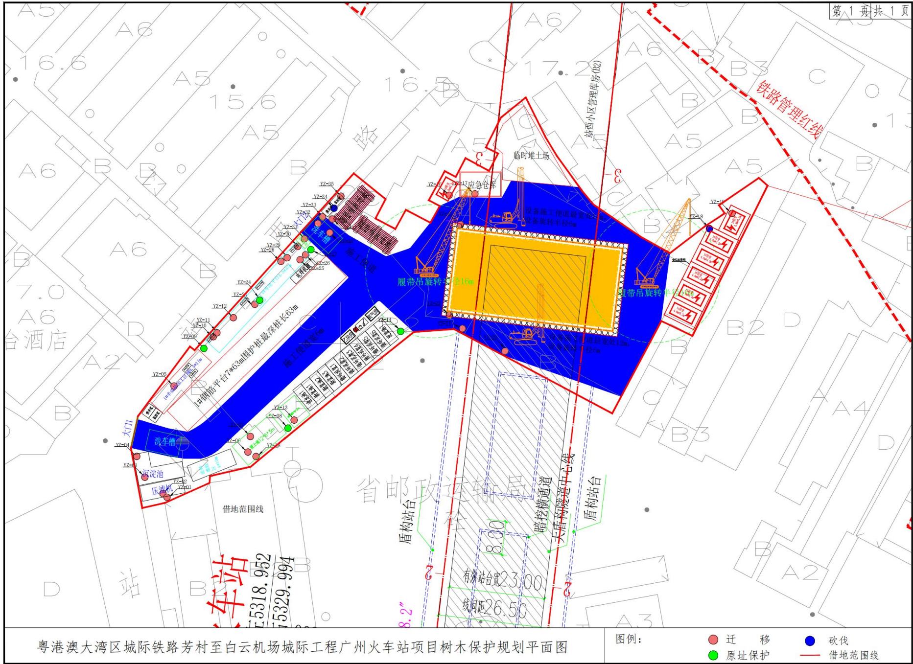
树木保护规划平面图:
