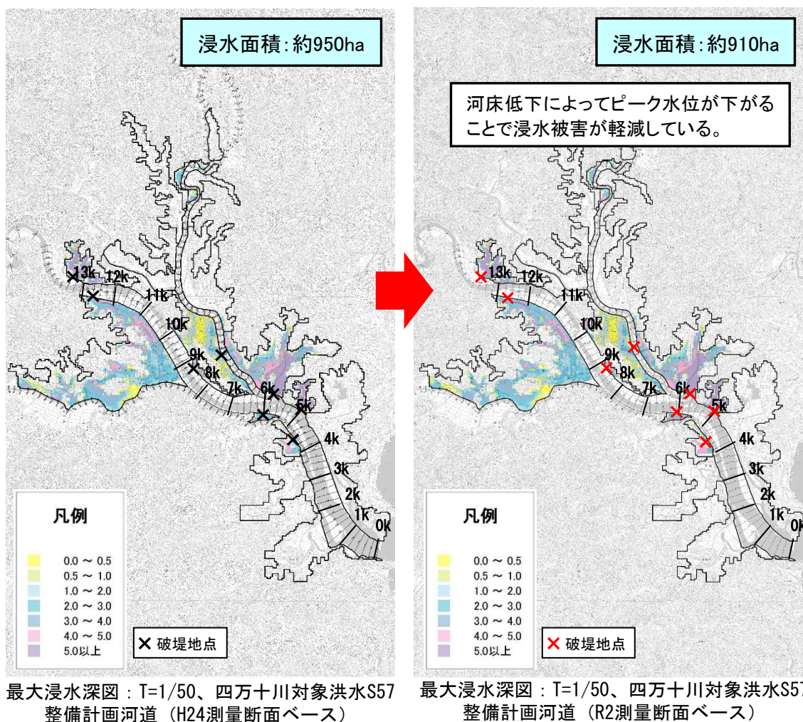
図 2.18 最大浸水深の比較（1/50 流量規模）
