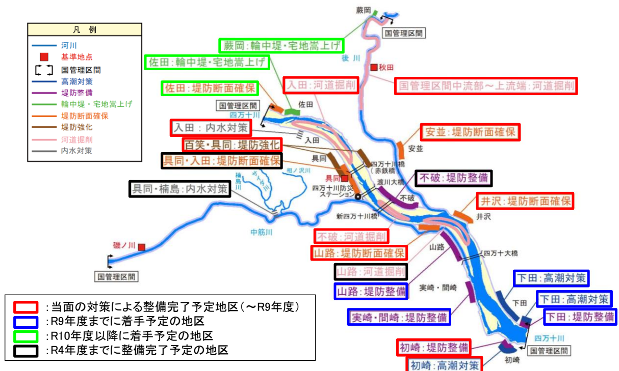
図 3.6 事業箇所位置図（当面の対策）
