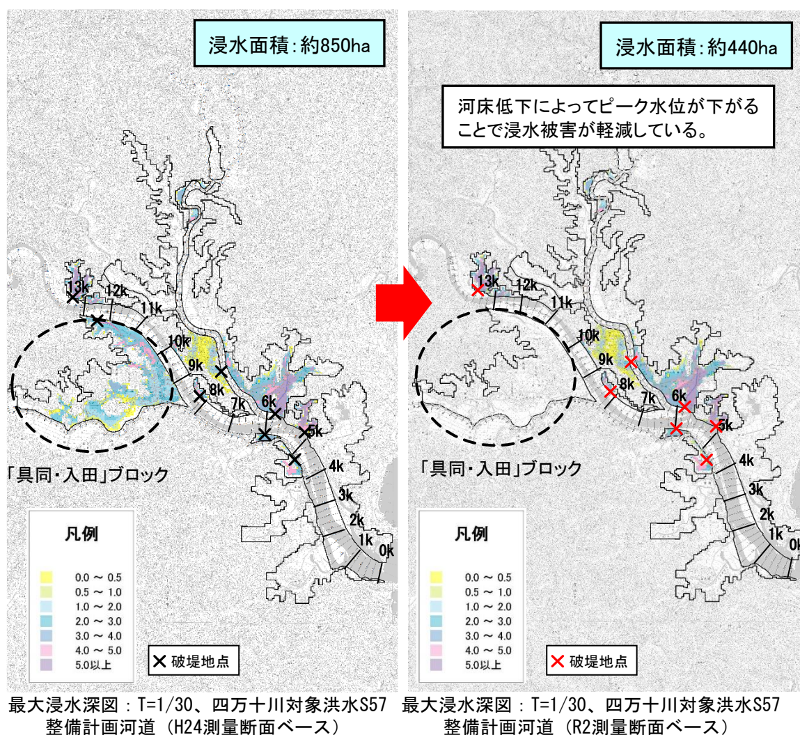
図 2.20 最大浸水深の比較 (1/30 流量規模)
