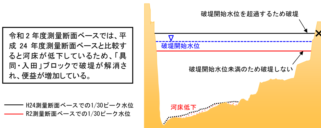
図 2.19 「具同・入田」ブロックにおける 1/30 流量規模のイメージ
