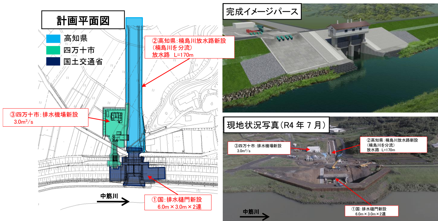
図 2.23 相ノ沢川流域の内水対策事業（楠島地区における楠島川放水路関連工事）
