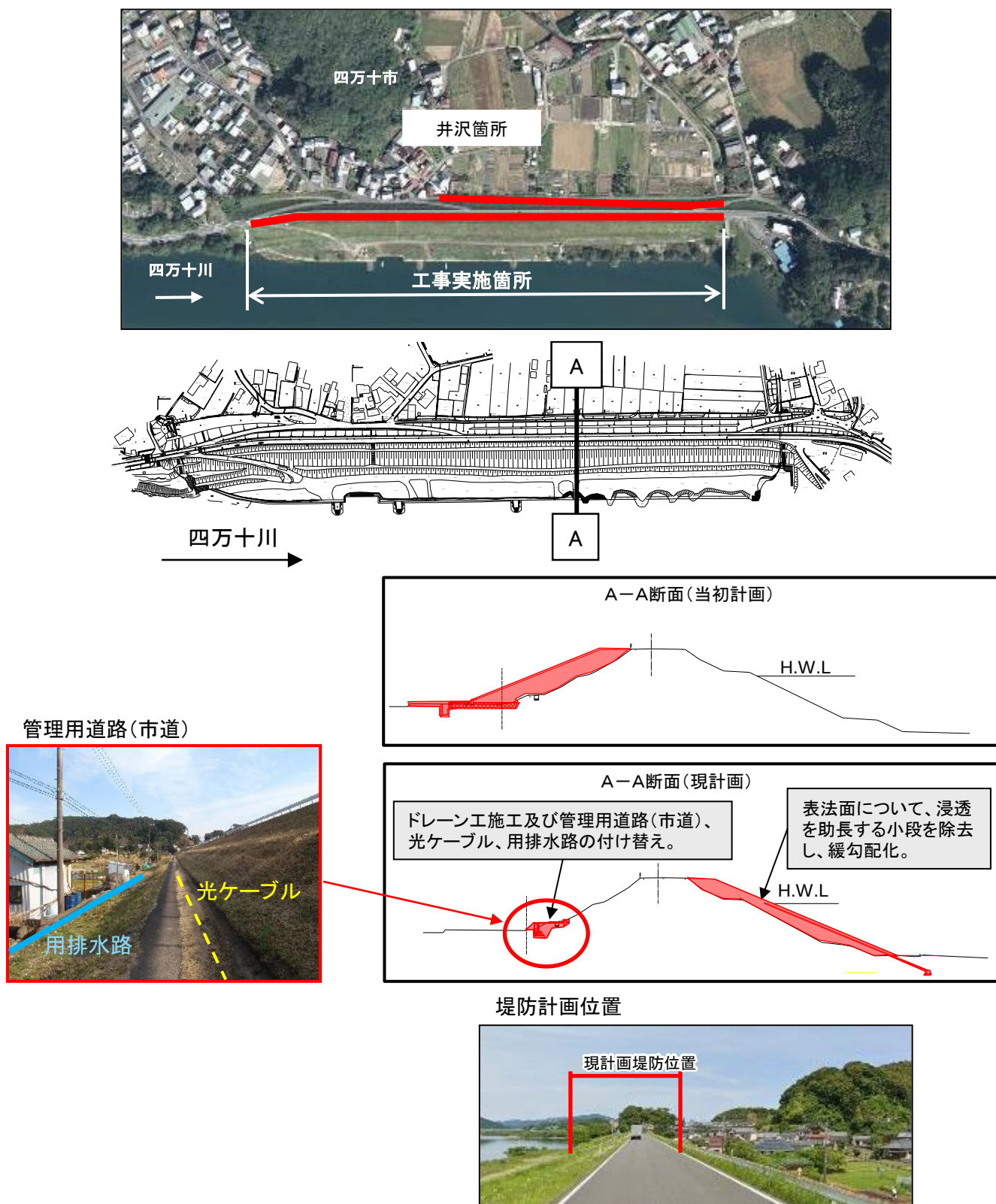
図 3.2 対策内容の精査に伴う計画変更
