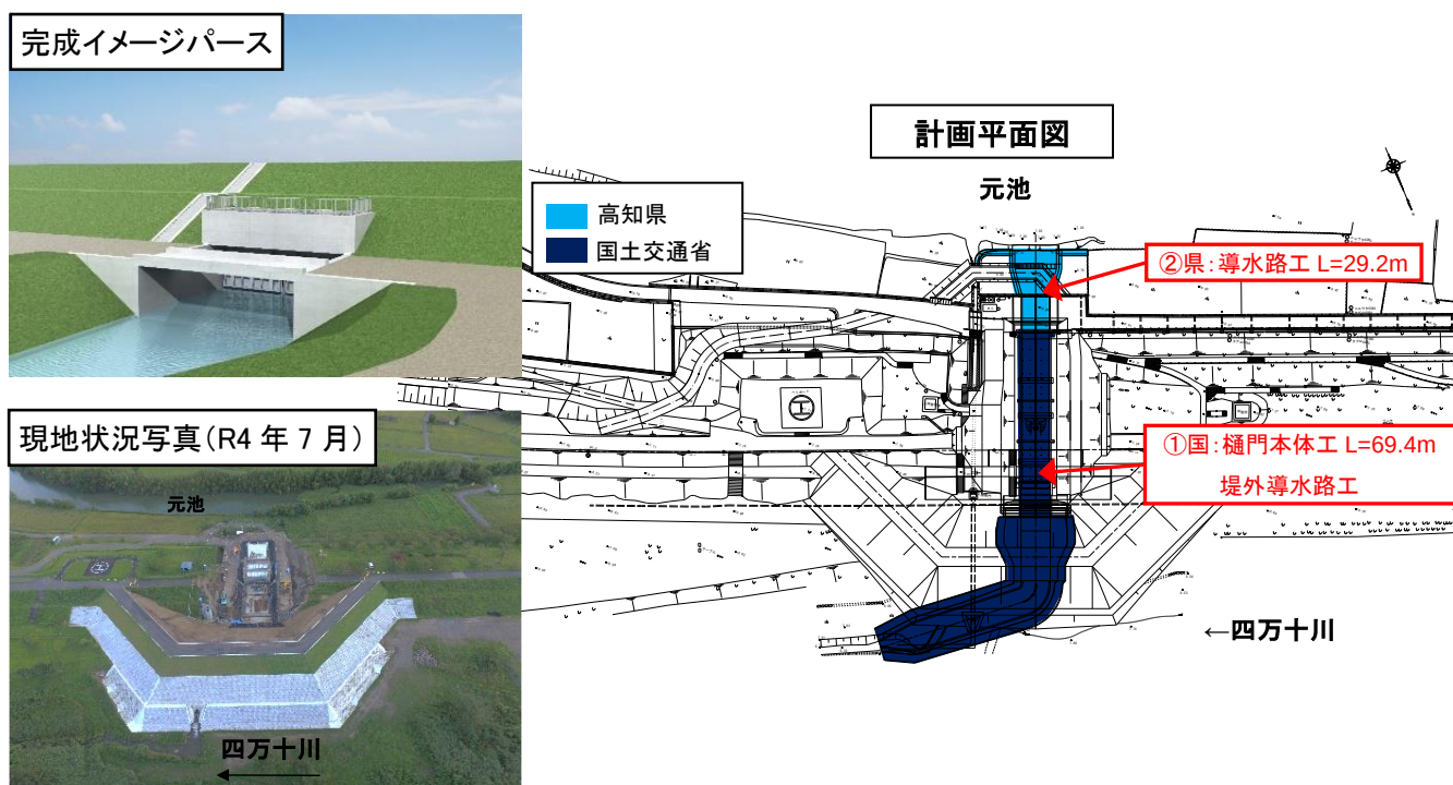
図 2.24 入田地区の内水対策事業
