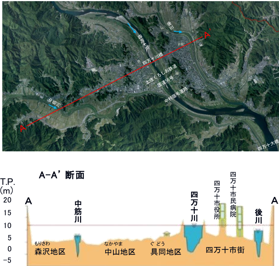
図 2.1 四万十川の沿川地盤高と計画高水位との関係（A-A' 断面）
