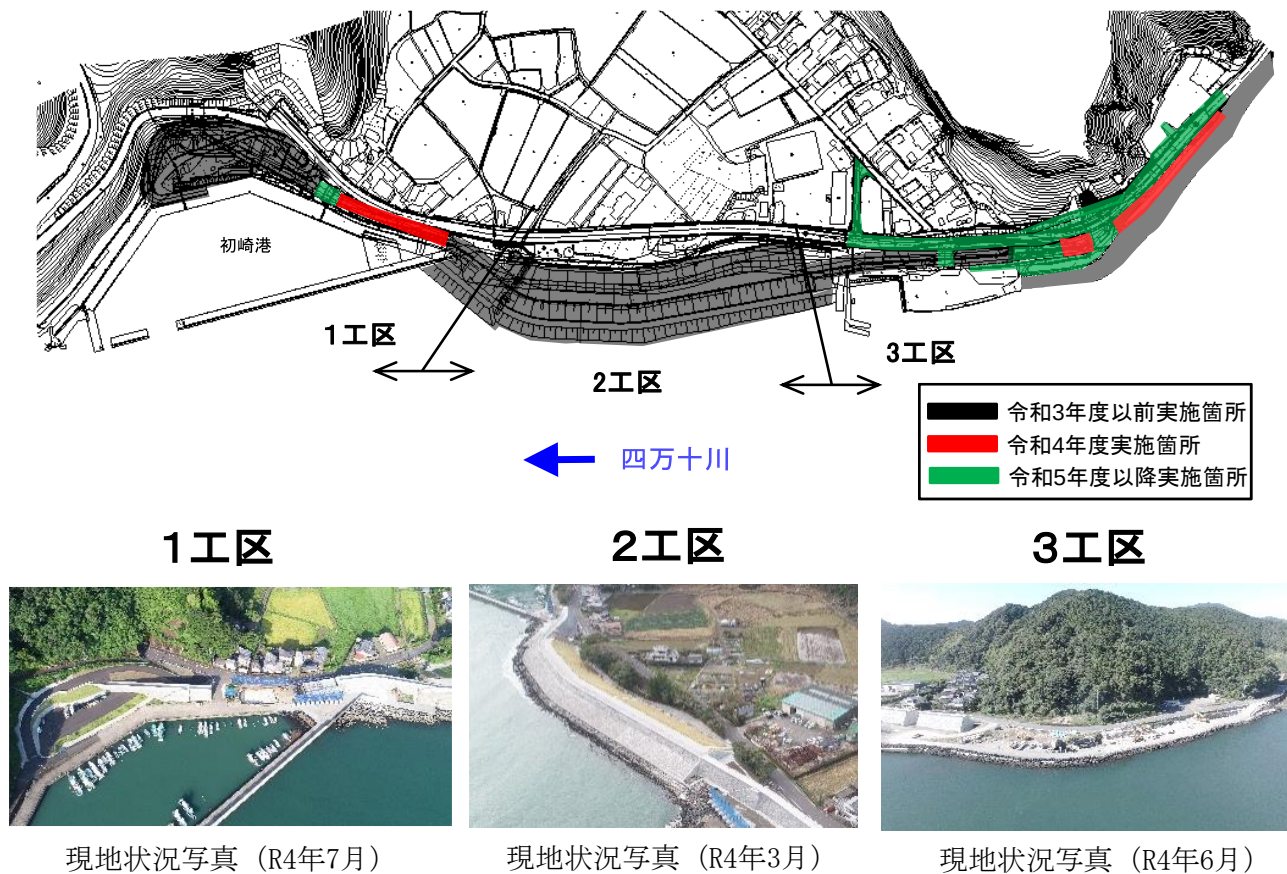
図 2.22 初崎地区の築堤事業
