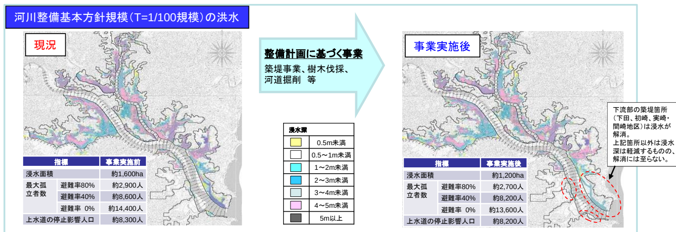
図 5.2 最大浸水深の変化（河川整備基本方針規模（T=1/100 規模））
