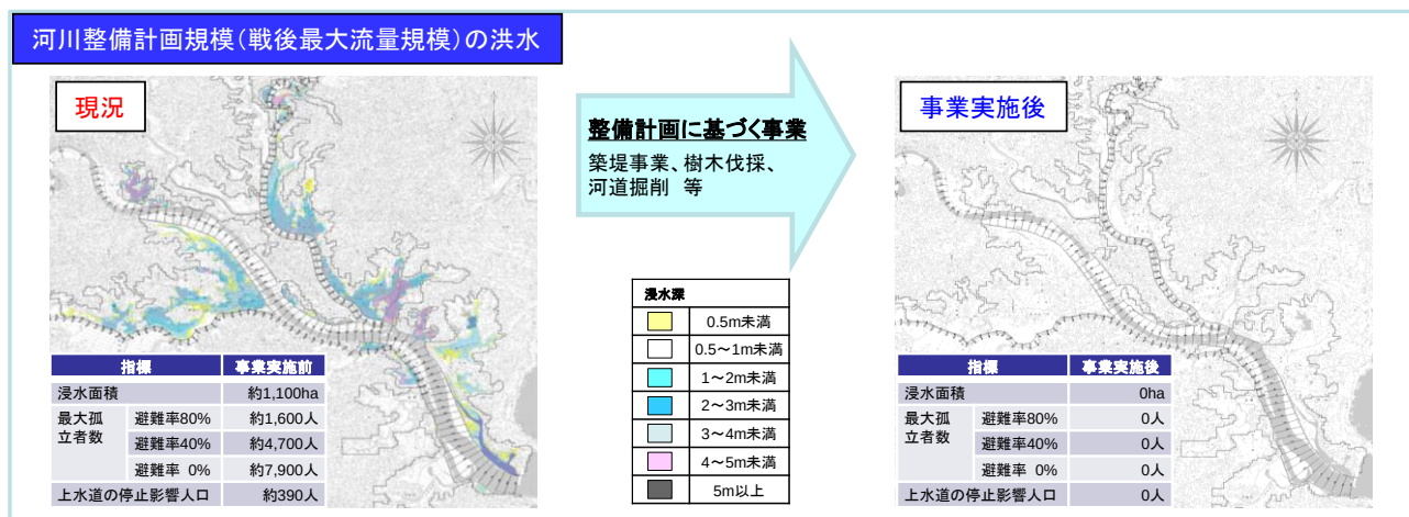
図 5.1 最大浸水深の変化（河川整備計画規模（戦後最大流量規模））
