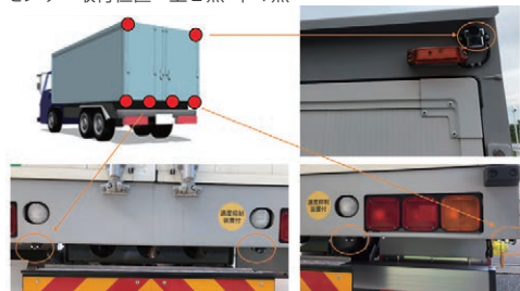
センサー取付位置：上2点・下4点
