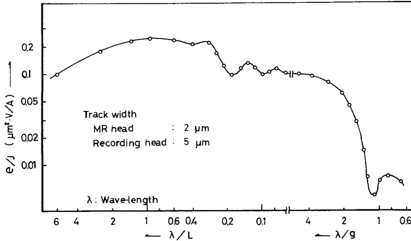
第 6 - 35 図 超狭トラック MR ヘッドの波長応答特性
