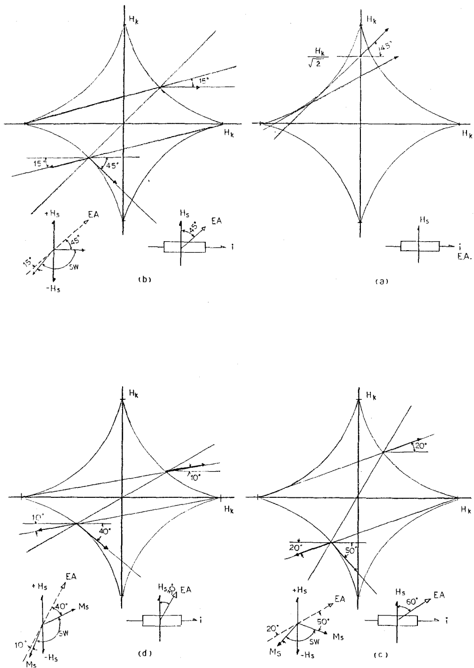
第6-2図 MR素子配向方向と磁化方向の関係を示すアステロイド曲線で示す図
