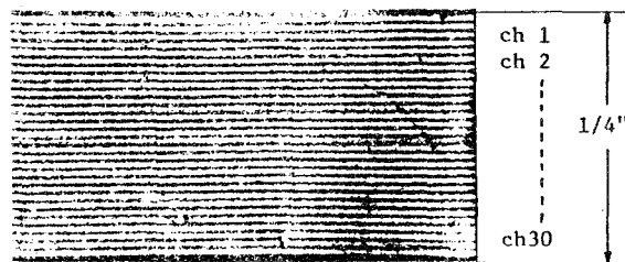
第4-25図 \frac{1}{4} インチテープ幅に30トラック記録した軌跡 ビッター現像図
