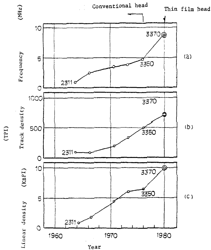
第7-1図 IBMタイプ記憶装置の進歩
