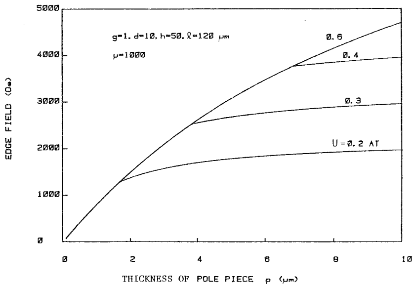
第 5-16 図 磁性層厚とギャップ端磁界との関係
