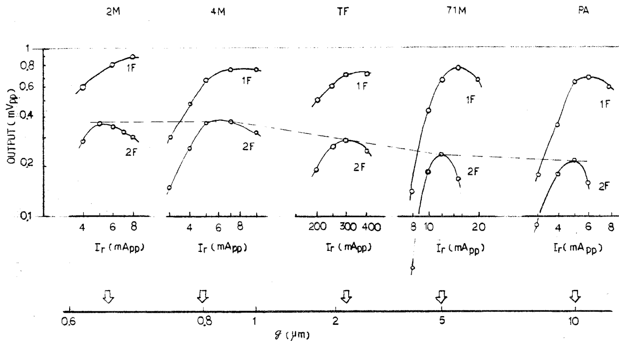
第4-13図 記録ヘッド・ギャップ長と入出力特性
