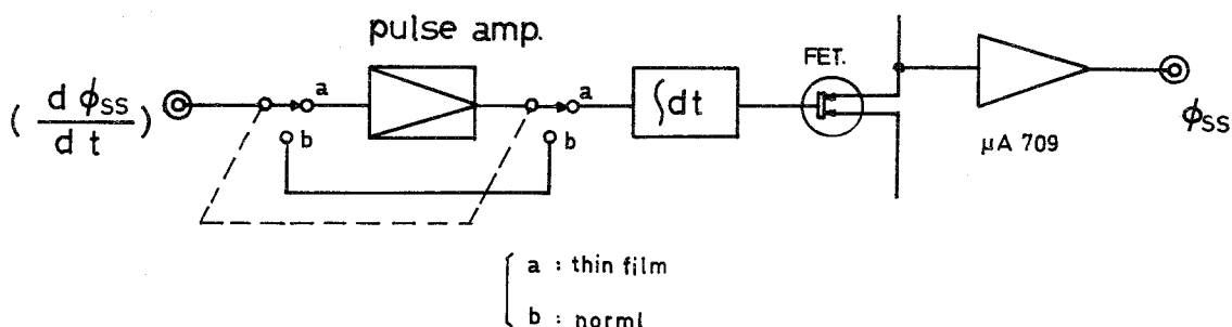
第3-10図 測定装置の電気回路系統図
