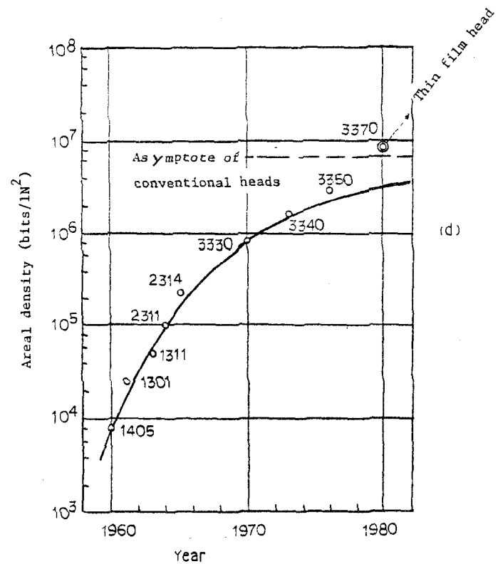
第7-1図 IBMタイプ記憶装置の進歩
