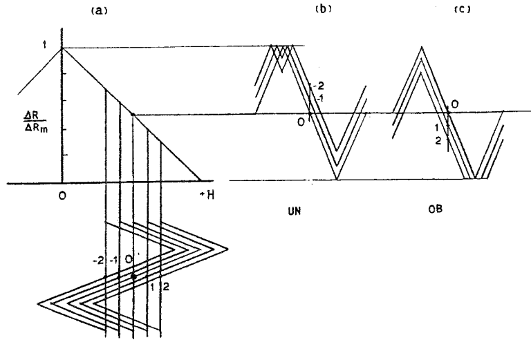
第6-4図 MR素子動作点のバイアス磁界による変化と信号磁界による抵抗変化
