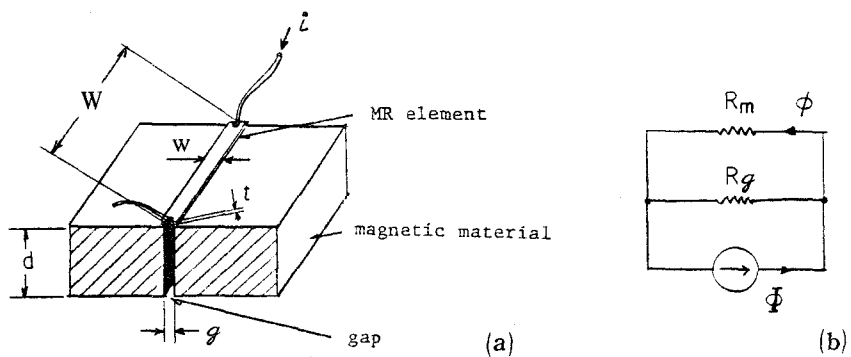
第6-25図 間接型MRヘッドの構造と磁気等価回路
