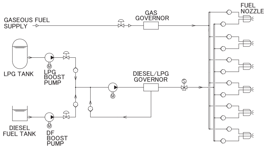
図1 トリプルフェューエル焼きシステムの燃料系統例
