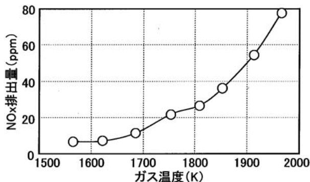
図17 モデルバーナのNO x 排出特性
