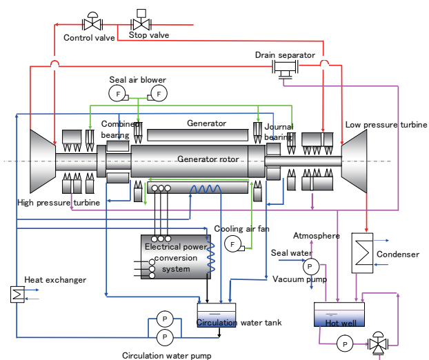
図1 タービンシステムの系統図
