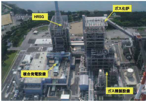
図7 IGCC実証機の全景
