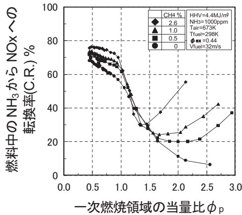
図8 一次当量比と燃料中NH 3 のNO x への転換率に及ぼす燃料中CH 4 濃度の影響（小型バーナを用いた実験結果）
