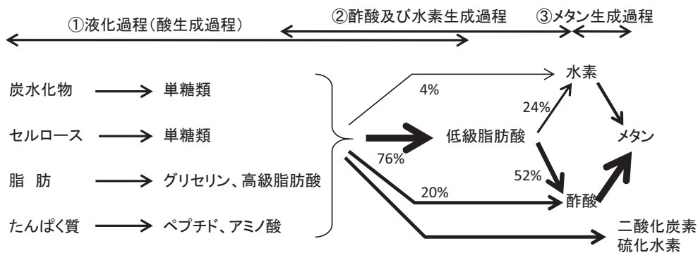
図2 メタン発酵のメカニズム
