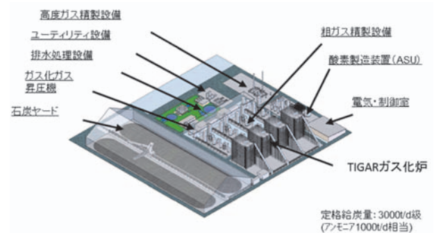
図11 アンモニア製造用ガス化プラント
