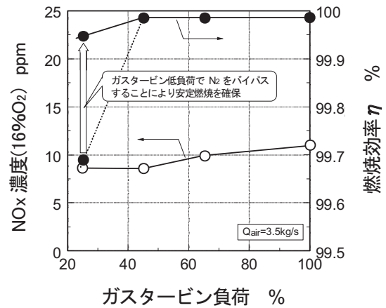
図12 湿式ガス精製対応型燃焼器の排出ガス特性
