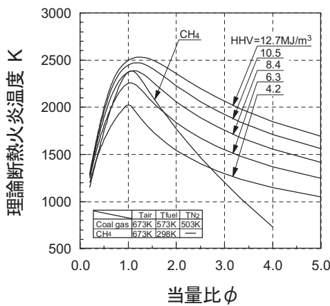
図 6 ガス化燃料および CH 4 の理論断熱火炎温度
