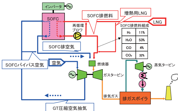
図11 トリプルコンバインドサイクル概略システム
