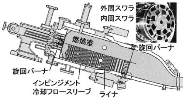
図11 空気吹きIGCC燃焼器構造
