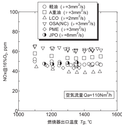
図3 NOx特性：燃焼負荷への依存性
