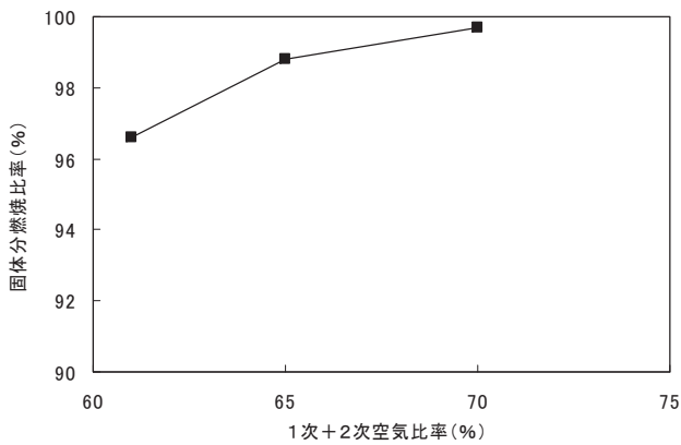
図6 空気配分と固体分燃焼比率の関係
