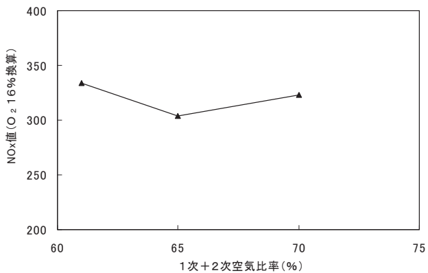
図7 空気配分とNOxの関係
