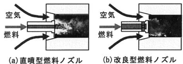
図5 クラスタバーナの混合可視化例
