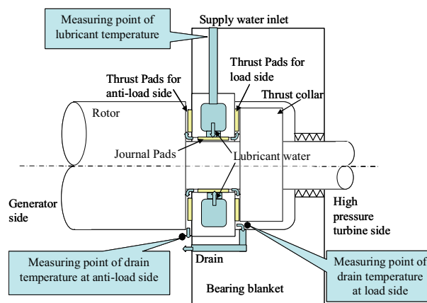
図10 コンバインド軸受の構造
