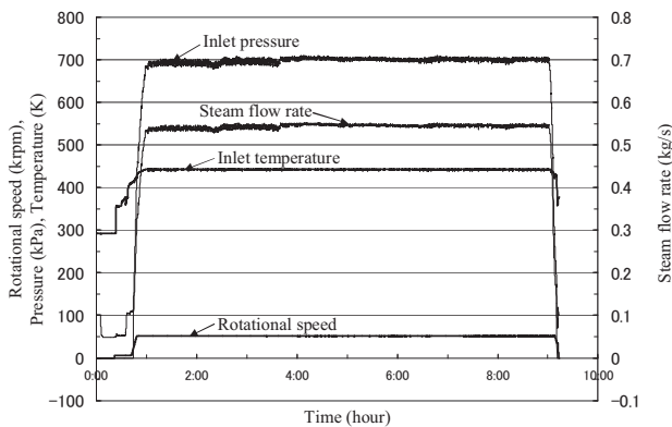
図12 高圧タービンの測定結果
