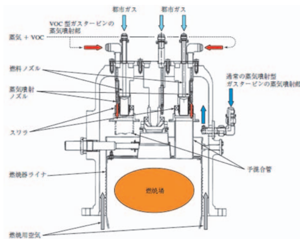
図1 VOC混焼DLE燃焼器 (IM270)
