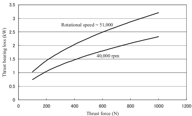
図7 スラスト軸受損失
