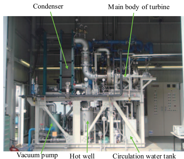
図8 プロト機の概観
