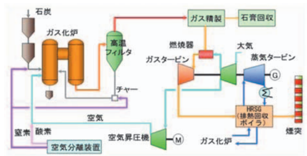
図6 石炭ガス化 (空気吹き) IGCCの概略系統図
