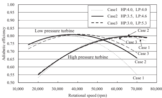
図3 タービン断熱効率
