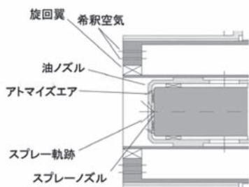
図1 バーナ断面図
