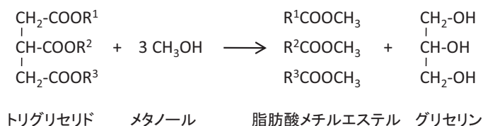
図4 エステル交換反応によるバイオディーゼル燃料の製造
