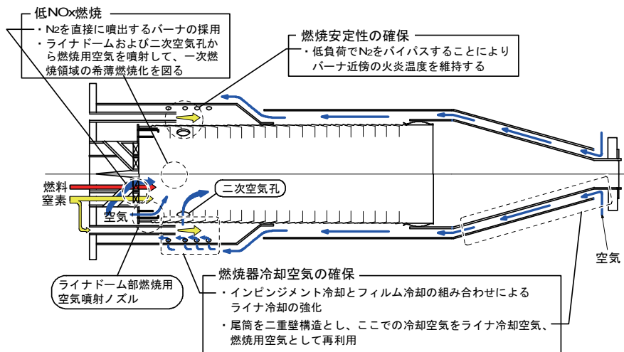
図11 湿式ガス精製対応型中カロリー燃料用ガスタービン燃焼器の概略
