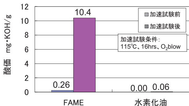
図4 水素化油の酸化安定性評価
