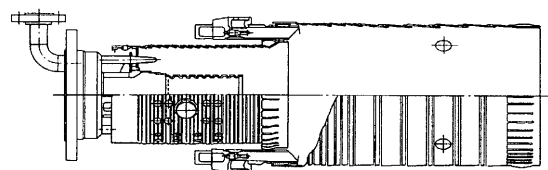
図5 フェーズI 燃焼器構造図
