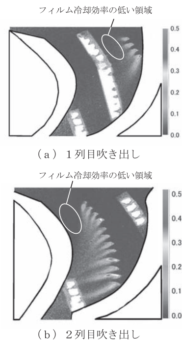
図16 プラットフォーム面のフィルム冷却効率コンター図
