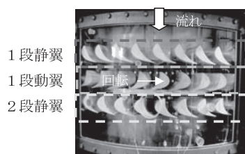
(b) 翼列部
