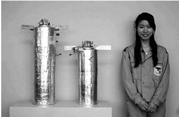
図5 一体型燃料処理装置の外観 (写真左は旧モデル、右は新モデル)
