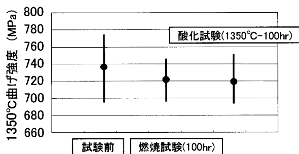
図16 セラミックの強度試験結果
