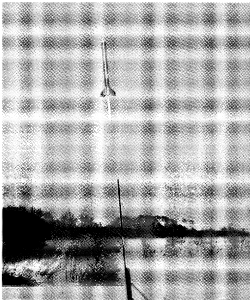
図4 酸化剤旋回流型ハイブリッドロケットの打上げ時の様子：2001年3月、北海道大樹町
