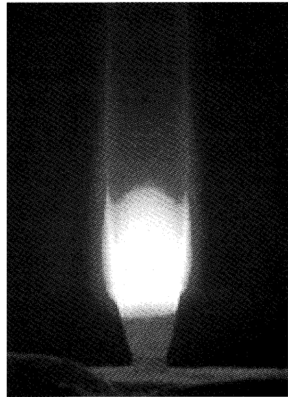
図6 二酸化炭素雰囲気中におけるMg蒸気噴流火炎：圧力35kPa、噴射管出口噴出速度62m/s
