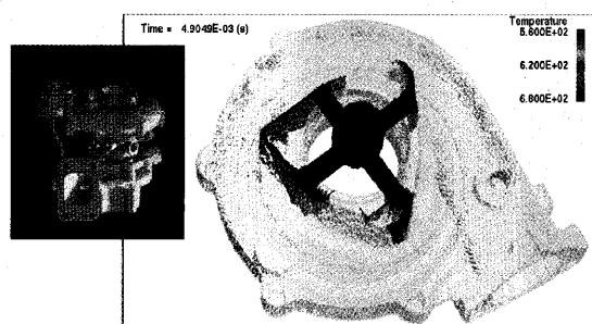
図4.6 CTデータからのボクセル解析(1) - 鋳造シミュレーション -
