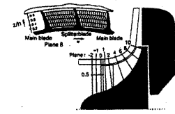
図5 Krain の LIFV による計測例 (3) と Hah の CFD 検証 (4)
