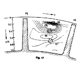
図5 Krain の LIFV による計測例 (3) と Hah の CFD 検証 (4)
