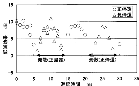
図8 燃焼騒音の低減効果と遅延時間との関係（メタン）
