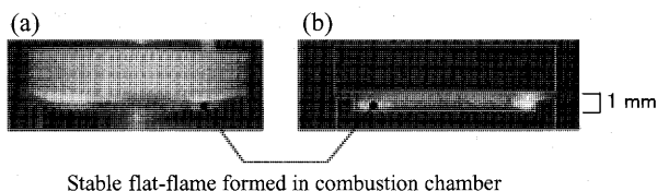
Fig.4 燃焼室内に形成された火炎のようす ( m_a=0.037\text{g/s} , \phi=0.4 ) (a)直接写真(露光時間180秒) (b)イメージインテンシファイアと CCD カメラ(露光時間1/30秒)
