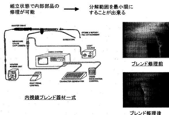
図7 動静翼の内視鏡ブレード修理
