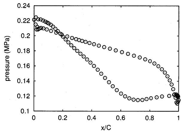
図7 99%スパンでの翼表面圧力分布 ( \phi 4 , 0%cl, adiabatic, U/C_0 = 0.6 )
