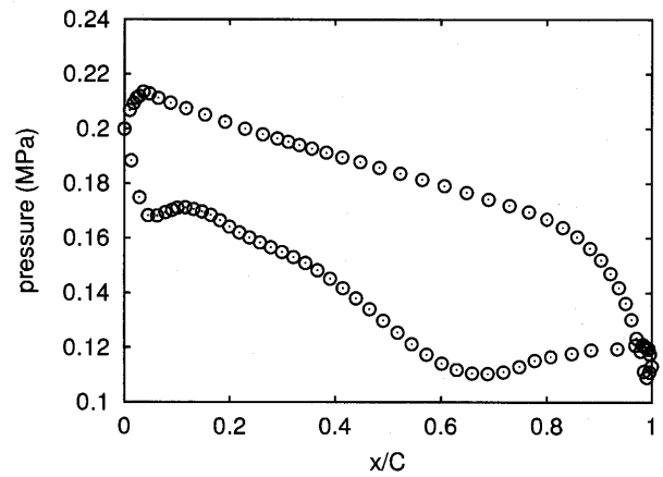
図6 94%スパンでの翼表面圧力分布 ( \phi 4 , 0%cl, adiabatic, U/C_0 = 0.6 )
