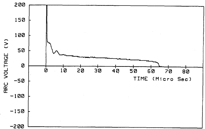
図6(a) スパーク電圧
