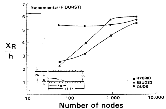
図 5.12 格子数と精度の比較 9)
