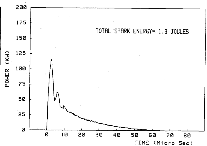
図6(c) スパーク電力
