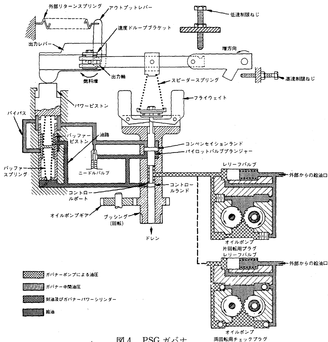
図4 PSG ガバナ
