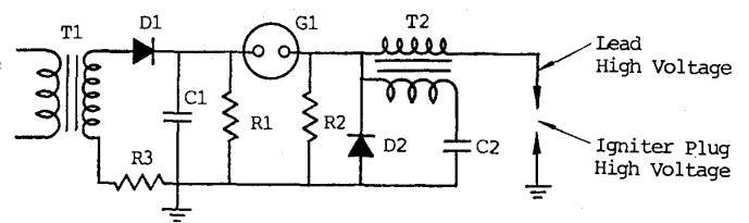
図4 高電圧容量放電型（単一極性回路）
