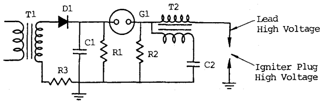
図3 高電圧容量放電型（振動回路）
