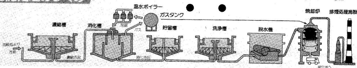
図2 下水処理／汚泥処理の概略
