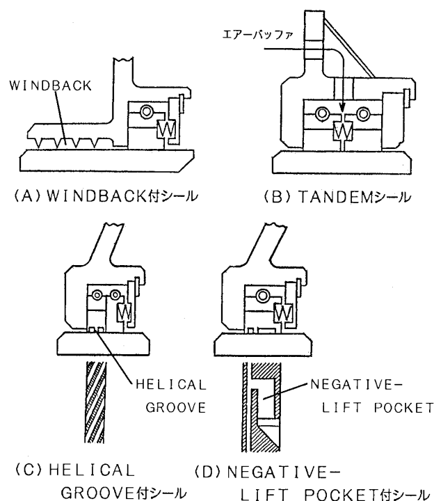
図5 オイルリーク対策用セグメントシール
