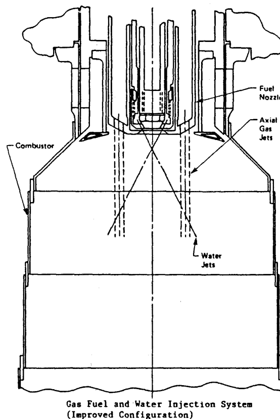
図 1.11 水噴射法 (ガス燃料, 産業用) 9)
