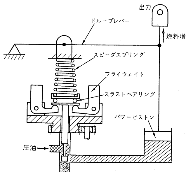
図3 SG ガバナ
