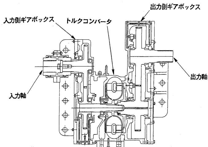
図2 500KW × 3000rpm
