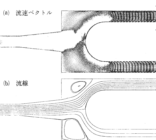
(a) 環状ダンプ・ディフューザの計算結果
