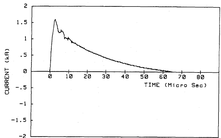
図6(b) スパーク電流
