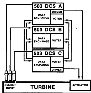
図11 503概念図
