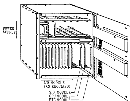
図10 501DCSの内部
