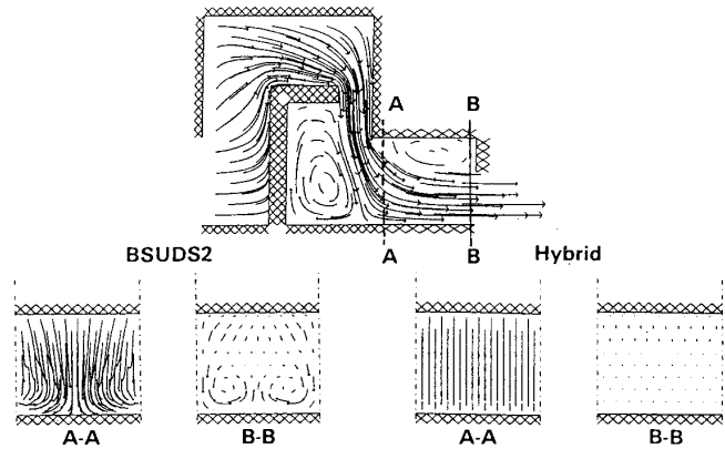
図 5.11 差分法によるフローパターンの解像度 9)
