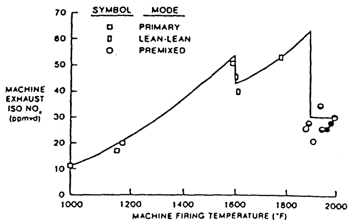
図 2.15 二段燃焼器(II)の \text{NO}_x 特性
