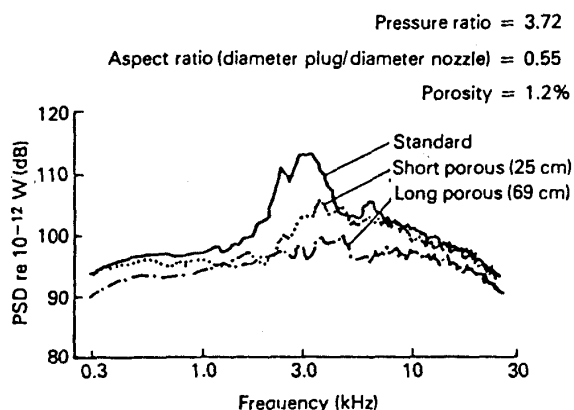
図 5.9 多孔プラグノズルと消音効果
