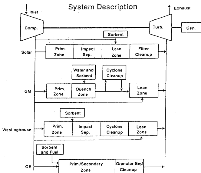
図 3.10 石炭焚ガスタービンのシステム
