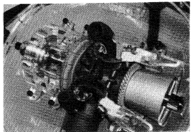
図3 乗用車用セラミックガスタービン (100 PS)
