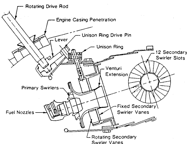
図2.24 可変機構付スワラ (Ⅱ.3.2の文献 3,17) )
