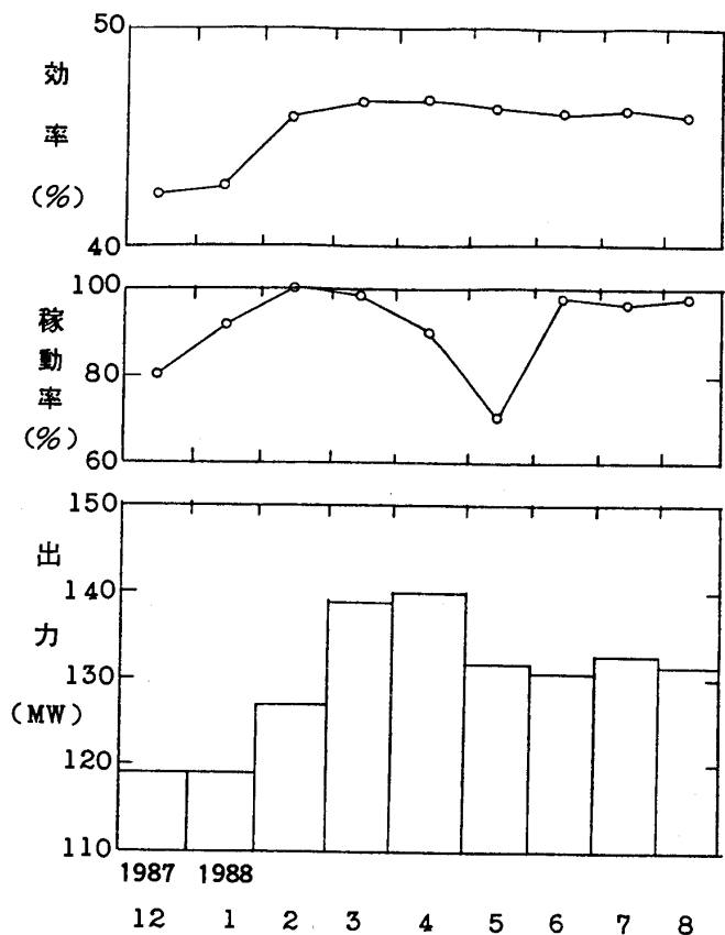
図4 稼働率と平均負荷
