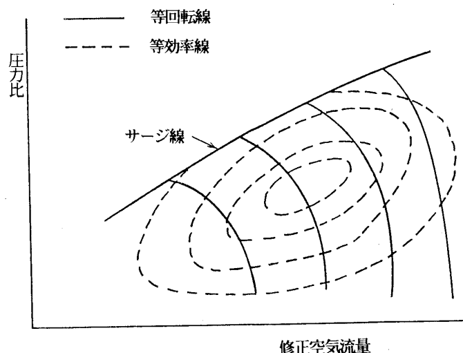
図 2 ファン及び圧縮機の特性マップの例
