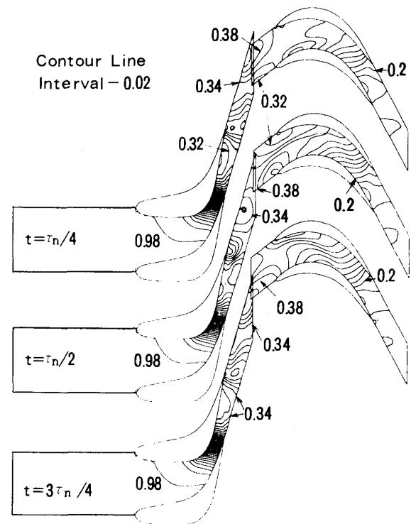
図11 等圧力線分布の時間変動
