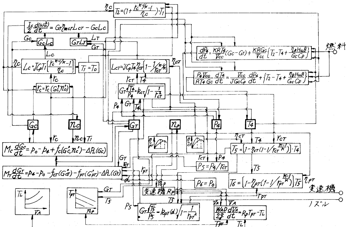
図2 2 質点モデルの情報流れ図
