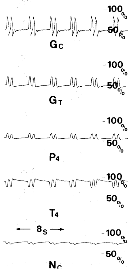
図10 ガスタービンのサージングの例
