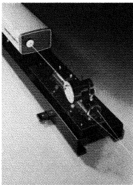
図11 後方乱方式によるアルゴン・イオン・レーザー流速計
