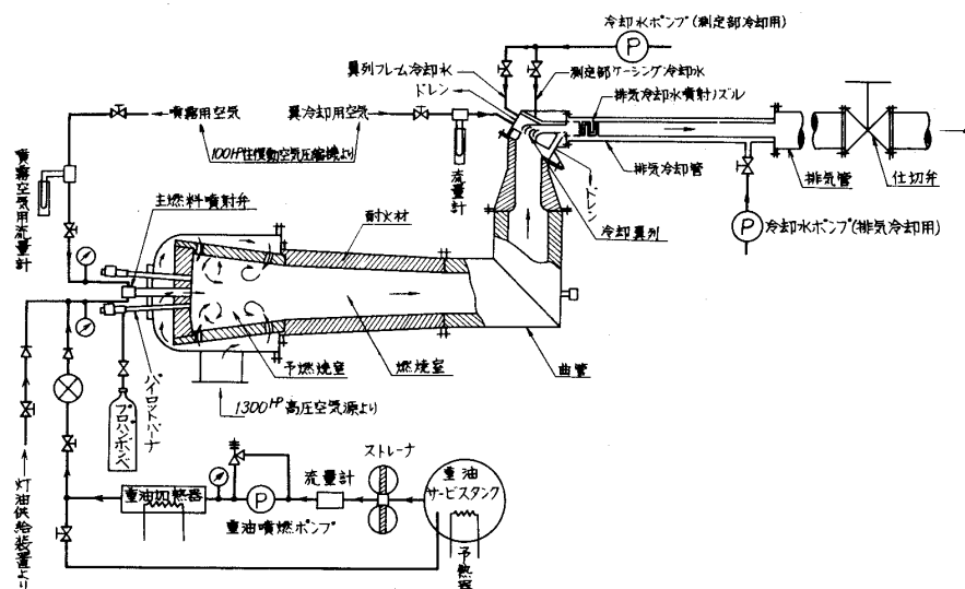
図1 実験装置
