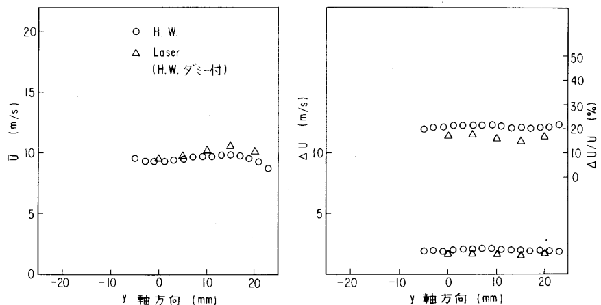
図10 熱線流速計との比較 (ブラフ・ボディ後方129mm)
