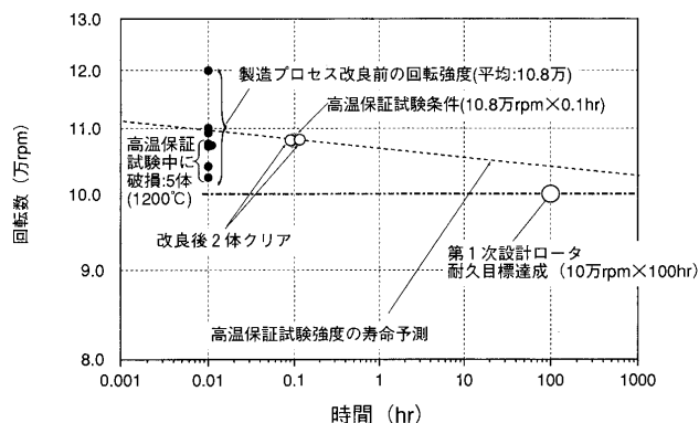
図 13 ロータ強度評価結果
