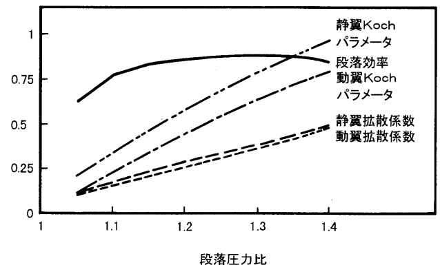
図8 段落圧力比の影響
