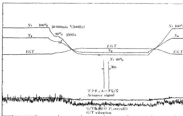
図6 100~60%回転速度可変試験
