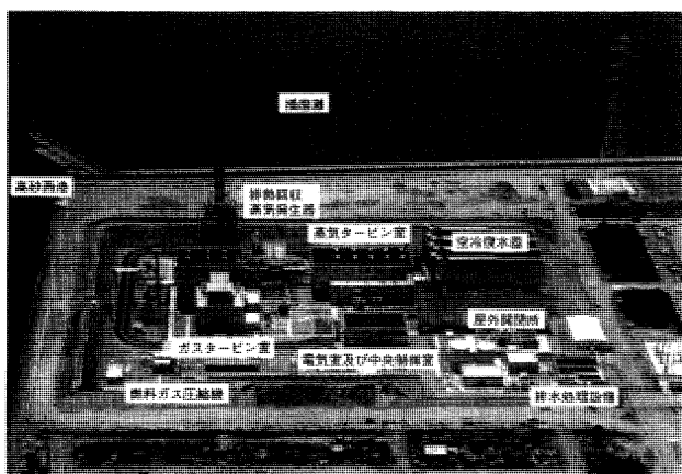
図7 三菱高砂製作所コンバインドプラント実証設備配置図
