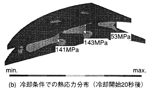
図 18 熱衝撃試験条件での応力分布
