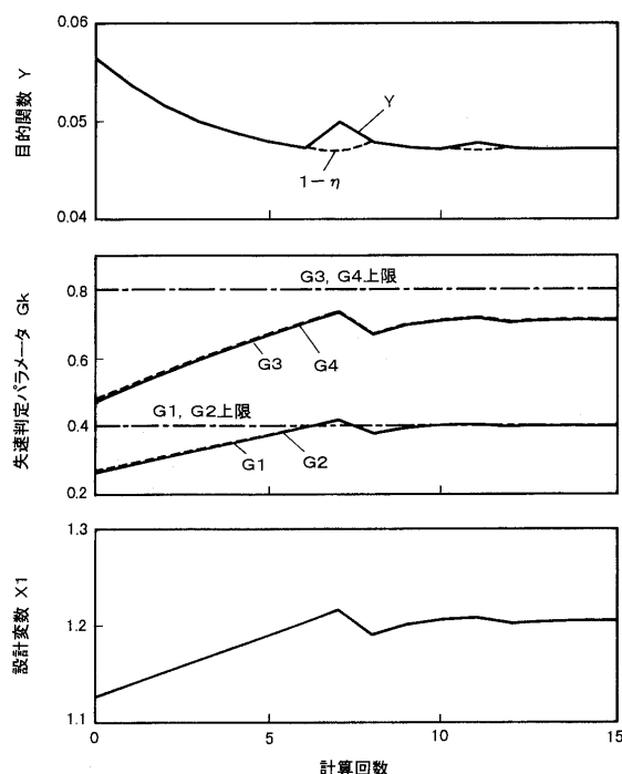
図 10 段落圧力比の最適化例
