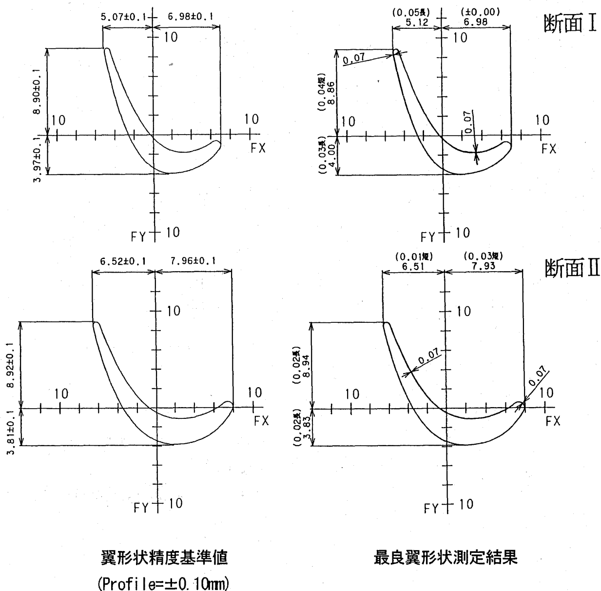
図2 Model-4 翼形状測定結果
