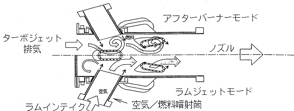
図2 アフターバーナー/ラム燃焼器作動図
