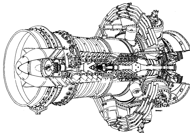
図 17 ドライ低 \text{NO}_x 燃焼器付き RB 211 (RR)
