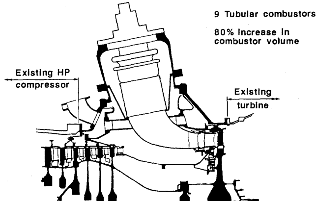
図 15 ドライ低 \text{NO}_x 燃焼器 (RR) (15)
