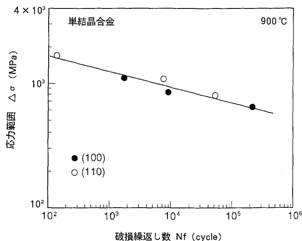
図4 単結晶材の低サイクル疲労強度 (応力範囲による評価)
