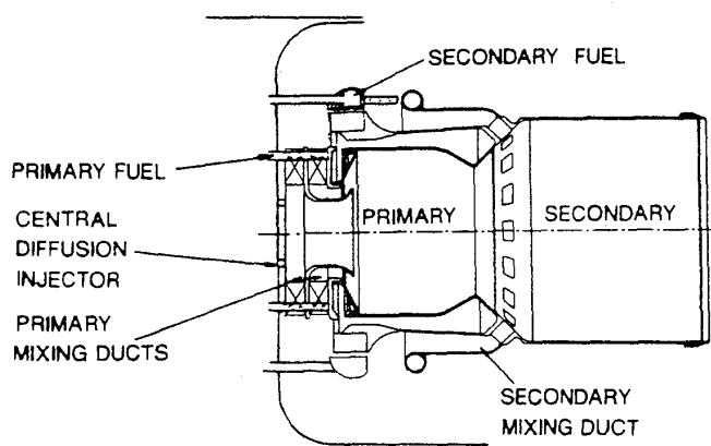
図 16 ドライ低 \text{NO}_x 燃焼器 (RR) (15)
