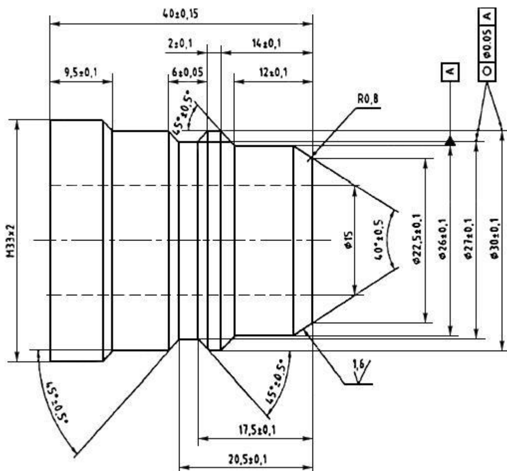
Рисунок Д.3 - Соединительный участок заправочного блока евро типа для АТС пассажирских и грузовых, имеющих максимальную общую массу менее 3500 кг
