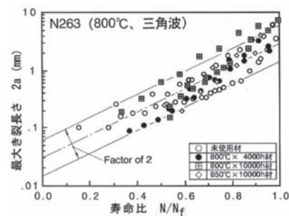
Fig.12 N263の最大き裂長さや寿命比の関係
