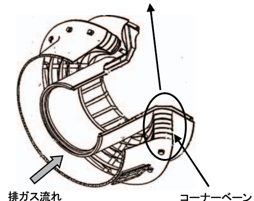
図6 E型排気ディフューザのき裂損傷状況
