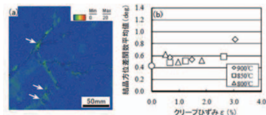
Fig.14 Ni合金クリープ模擬損傷材のEBSD分析例 (a)結晶方位差関数マップ、(b)クリープひずみと結晶方位差関数平均値の関係
