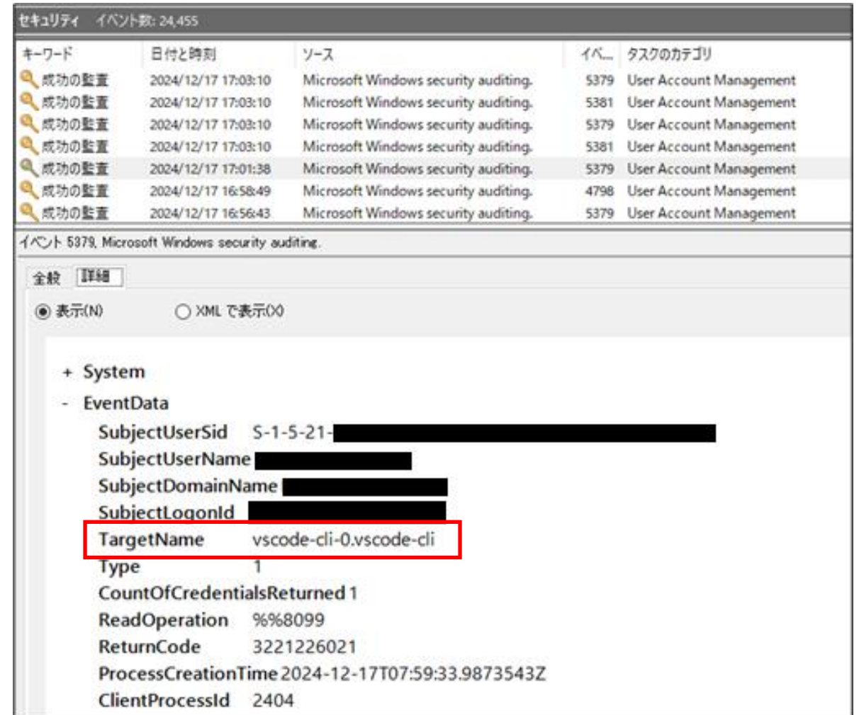
図3: イベントログ「Security」
