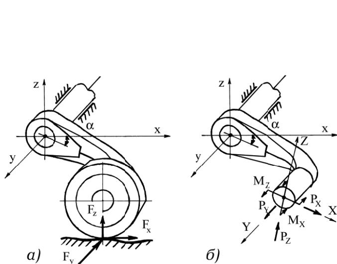
Рис. 8. Нагрузки, действующие на балансир
