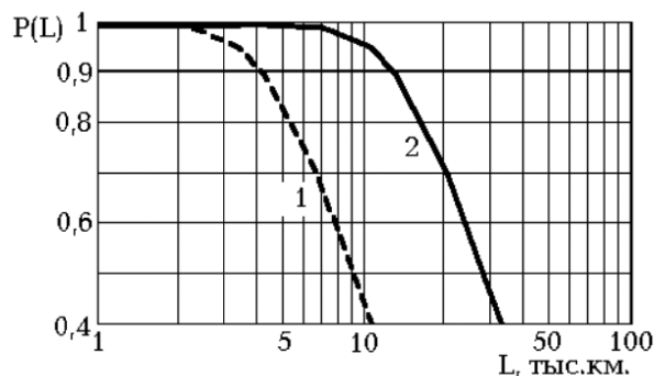
Рис. 10. Функции надежности балансира: 1 – исходный вариант; 2 – усиленный вариант конструкции
