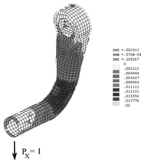
Рис. 9. Распределение напряжений в теле балансира
