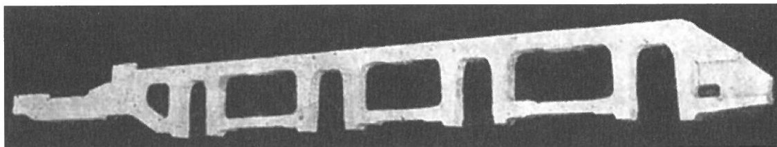
写真3 鉄道省蒸気機関車の鑄鋼製と思しき主台枠サイドメンバ
