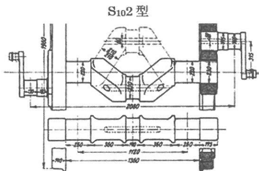
図12 プロイセン国鉄G 12 型およびS 102 型蒸気機関車の一体鍛造クランク車軸
