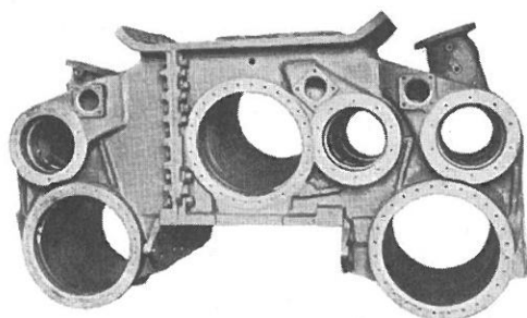
(a)初期の鋳鋼製2分割式(後方より)
