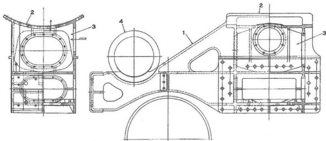
図3 C55型蒸気機関車の排気膨張室付き罐台と台枠への取付け状況
