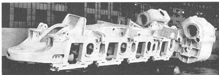
1DD1連節機関車の前部ユニット
