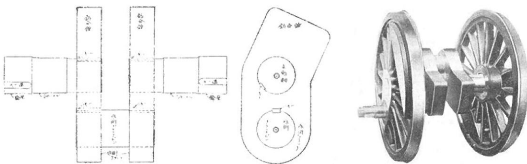
図13 / 写真5 C53の組立クランク車軸(改造後)鍛造クランク車軸
