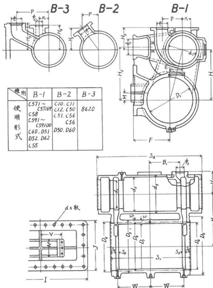
図4 排気膨張室付き罐台に対応する排気ツナギ管付きの気筒体
