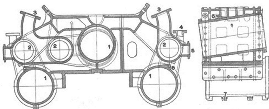
図1 C53の2分割気筒体(正面図は前方より)
