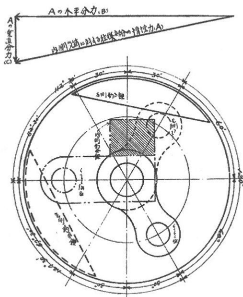
図6 C53の主動輪のクランクウェブに付加された釣合錘 (斜線部、改造前、右側より、西尾前掲書、143頁、第68図)
