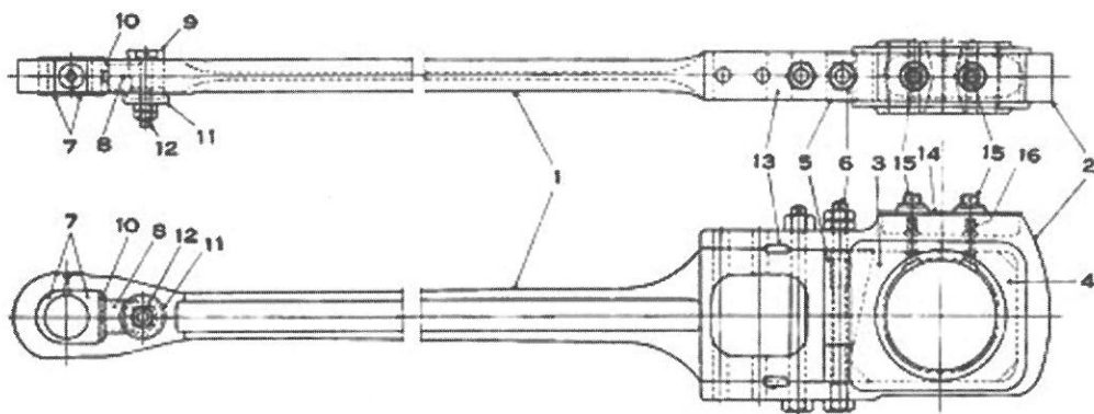
(a) C53の中央主連棒(中心間距離2700mm, 通常構造の太端を有する外側のそれは3100mm).
