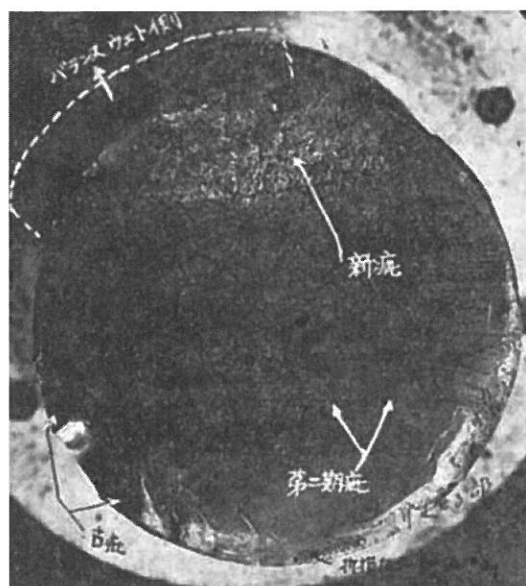
写真6 C5357における組立式クランク車軸の折損事例(左側軸頸)
