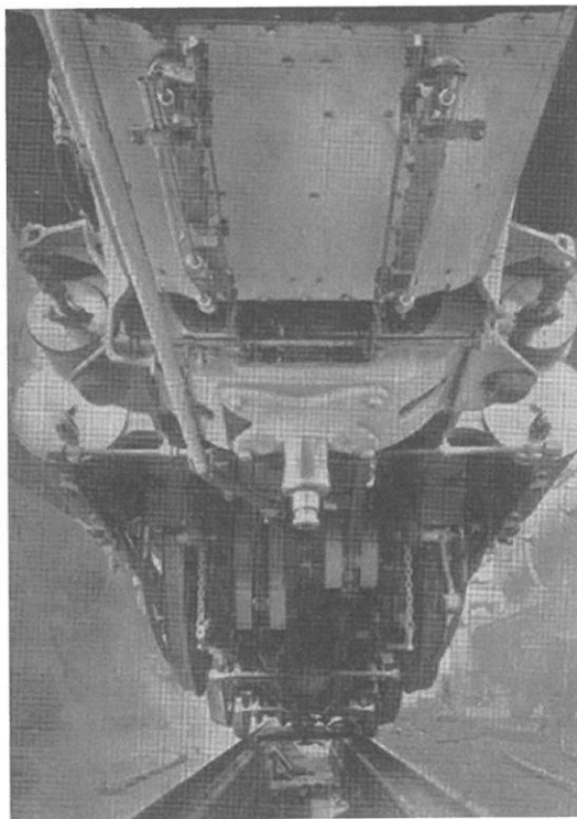
写真7 G.W.鉄道“King”級4気筒蒸気機関車の機関部
