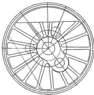
図7 C53の主動輪のクランクピン配置と釣合錘配置
