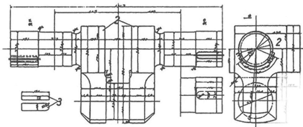
図11 C53初期の一体型クランク軸
