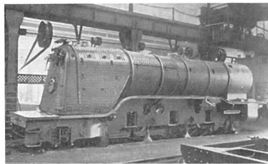
写真4 Gresleyパシフィック第1号機 A1 No.1470 Great Northernの建造風景
