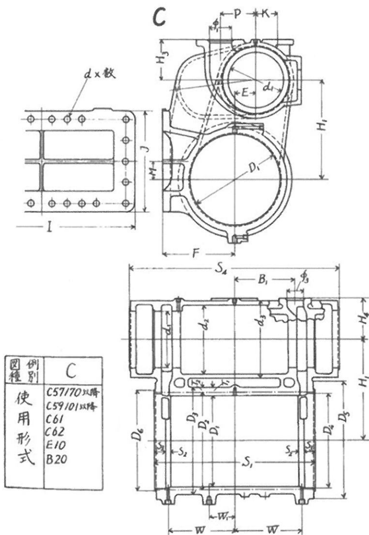
図5 排気ツナギ管なしの排気膨張室に対応する戦後の標準型気筒 (国鉄工作局動力車課監修『蒸気機関車各部設計寸法』9頁、より *10) )
