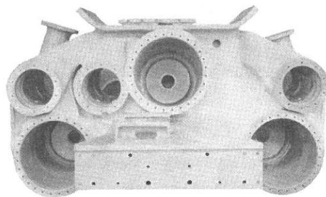
(b)後期の鋳鋼製一体式(前方より)
