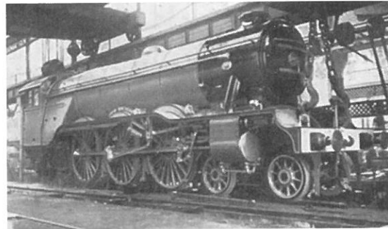
写真4 Gresleyパシフィック第1号機 A1 No.1470 Great Northernの建造風景
