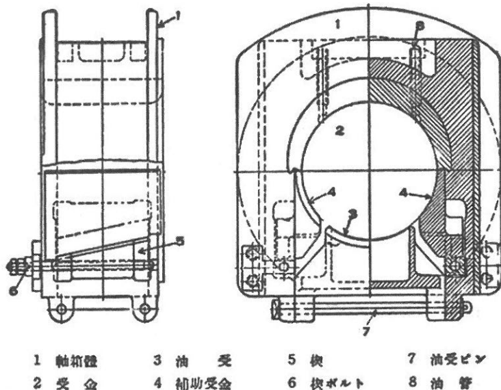
図10 C53の主動軸軸箱
