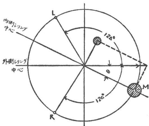
図8 C53設計に際して開発された主動軸回転質量釣合法 (機関車工学会『新訂増補 機関車の構造及理論』中巻、交友社、1941年、235頁、第162図より)
