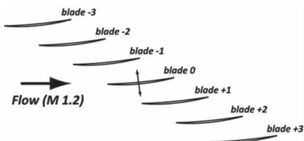
Fig. 1 Test cascade
