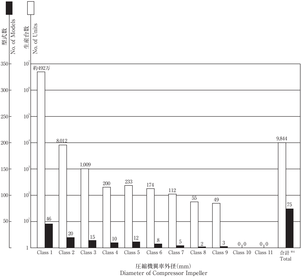
図11 2020年過給機生産台数及び型式数（注※4は表10を参照）
