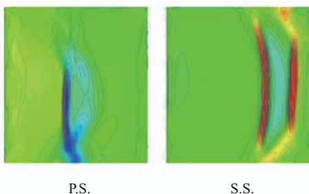
(d) Resultant W distribution on blade (CFD)
