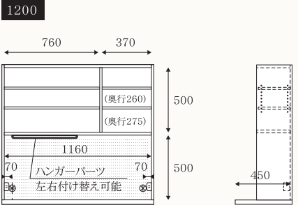
⑤⑥1200オープンガラス戸/板戸 W1200 / D465 / H1080 可動棚板:大2枚・小2枚
