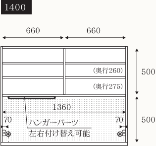
⑦⑧1400オープンガラス戸/板戸 W1400 / D465 / H1080 可動棚板:4枚
