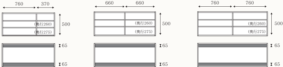
⑩1200吊り板戸 W1200 / D310 / H565 可動棚板:大2枚・小2枚
