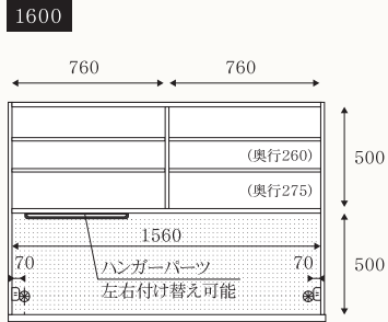
⑨⑩1600オープンガラス戸/板戸 W1600 / D465 / H1080 可動棚板:4枚
