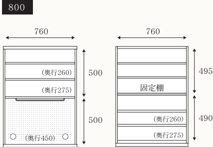
②800オープン板戸 W800 / D465 / H1080 可動棚板:2枚 ③④800ガラス戸/板戸 W800 / D465 / H1080 可動棚板:4枚
