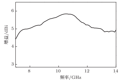
图10 天线增益
