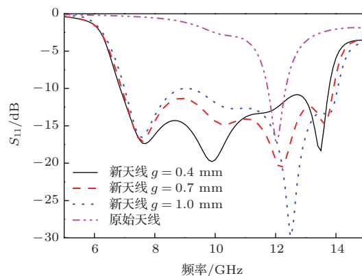
图3 (网刊彩色) 原始天线和新天线的比较
