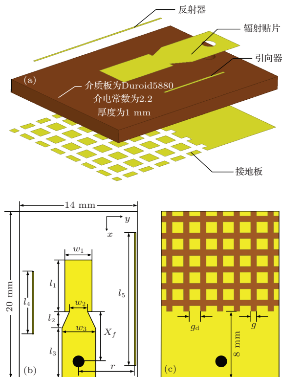
图1 天线结构图 (a) 三维视图; (b) 天线上表面; (c) 接地板
