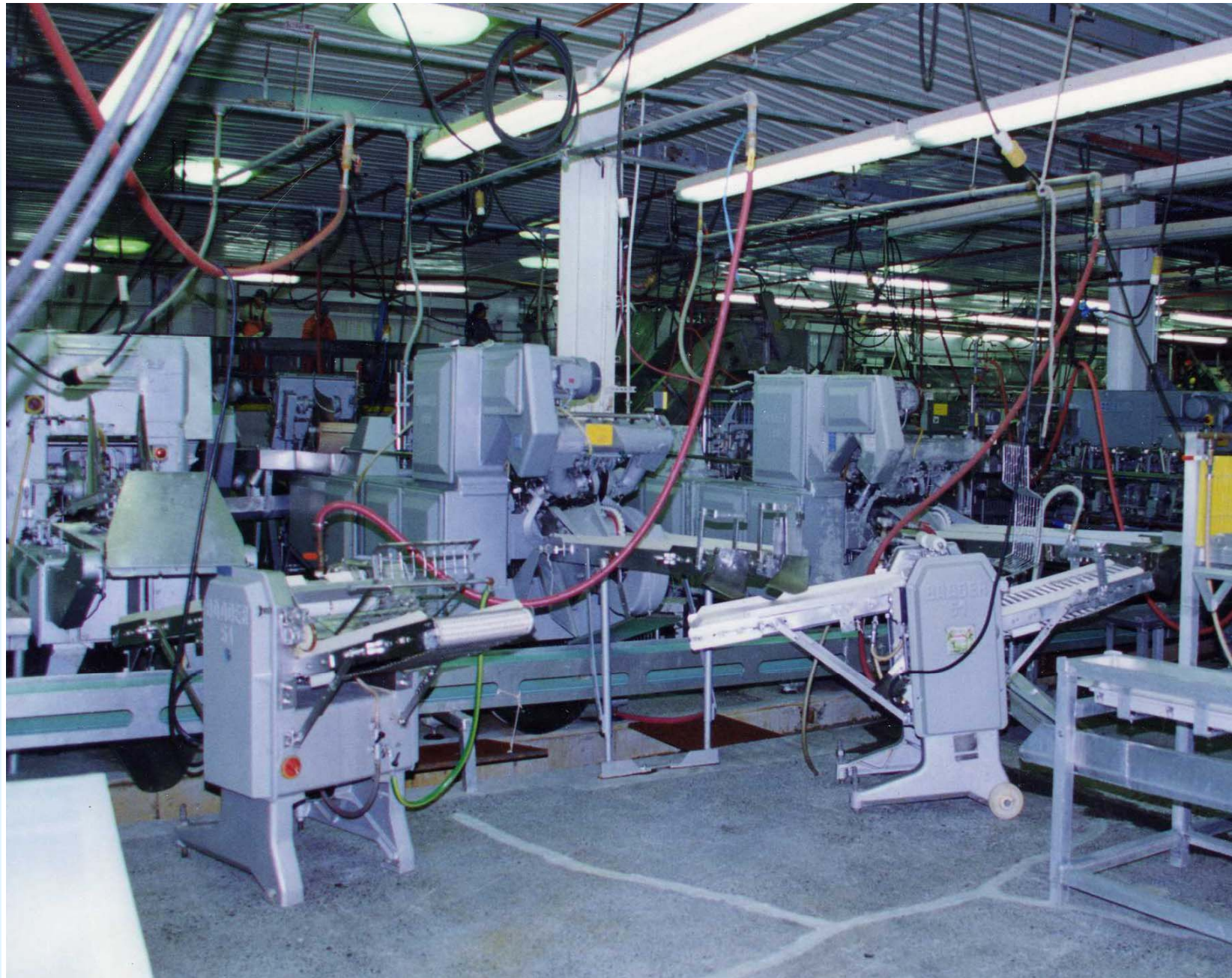
第二魚加工場内部（ポーラック・コッド・フラットフィッシュのフィレマシン 後にここにフィッシュパウダーマシンを装備してフィッシュパウダー生産を行なう）
