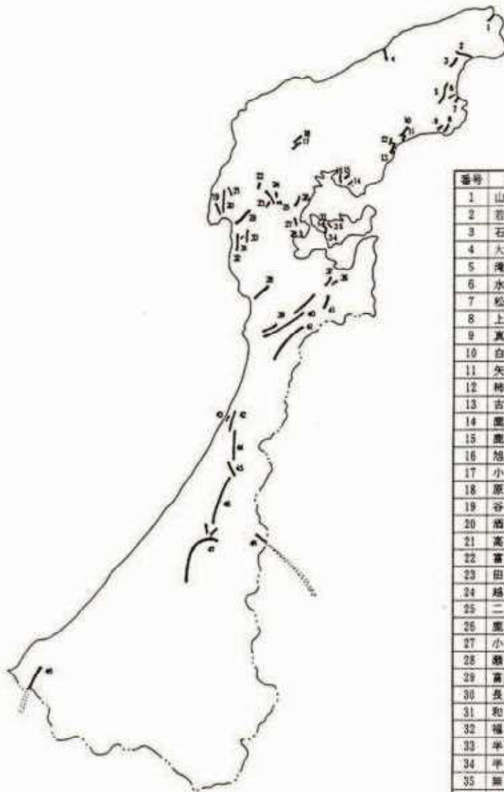
図 石川県の活断層
