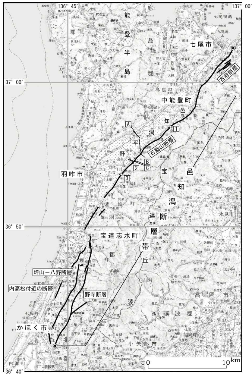
図 邑知潟断層帯の活断層位置図
