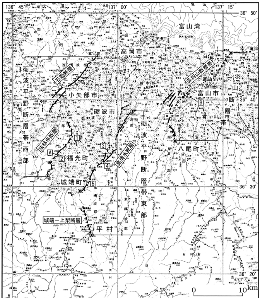
図 砺波平野断層帯・呉羽山断層帯の活断層位置図
