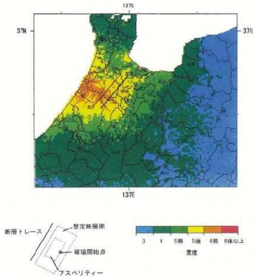
図 新波平野断層帯西部の後振動評価
