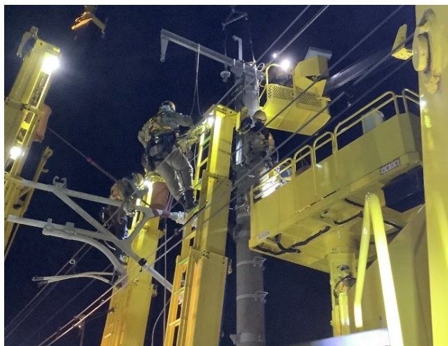
建柱車による電柱の鋼管柱化工事
