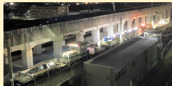
保守基地から施工場所に向かう大型機械
