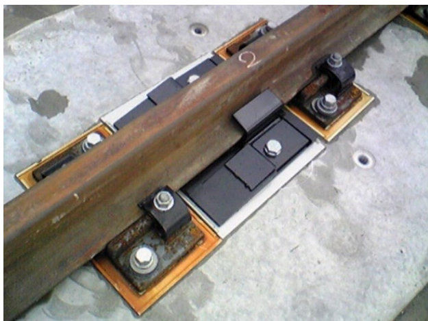
レール転倒防止装置の設置
