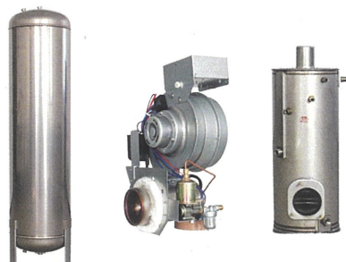
熱交換器(セミ貯湯タイプ)、ステンレス貯湯タンク、バーナー(ガンタイプ)
