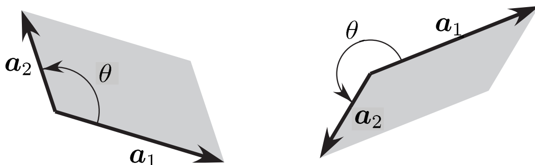
図 7.1 二つの二次元のベクトル \mathbf{a}_1, \mathbf{a}_2 のつくる平行四辺形。左では「符号付き面積」は灰色の平行四辺形の面積そのもの。右では \theta > \pi なので、「符号付き面積」は灰色の平行四辺形の面積にマイナスをつけたものとする。
