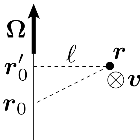
図 6.16 剛体上の点 r の速度 v と角速度 \Omega の関係 (6.4.15) を考えるための図。 \otimes という記号は、ベクトル v が紙のこちら側から向こう側にむかっていることを表す。こういう図は、本文を読みながら、自分なりに工夫して描いてみるのがもっともいいだろう。
