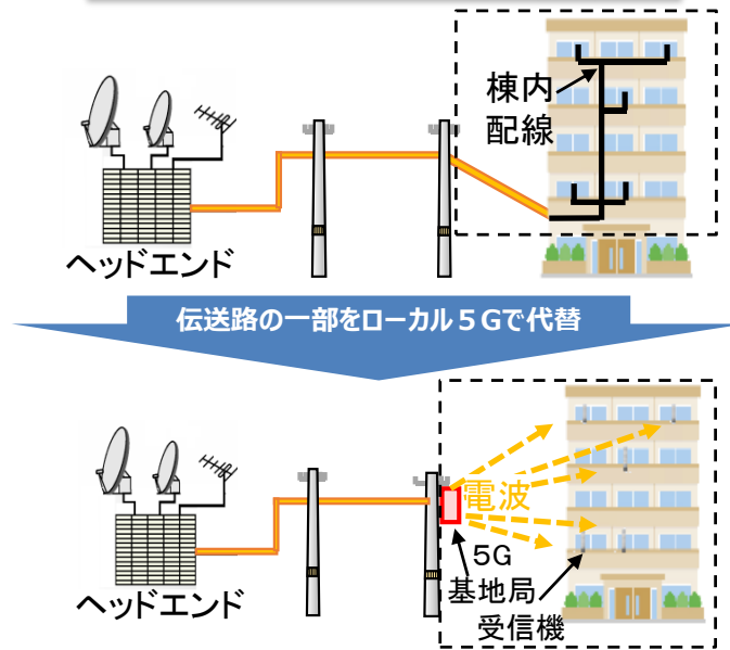
【図表 20 ローカル 5G を活用した改修イメージ】
