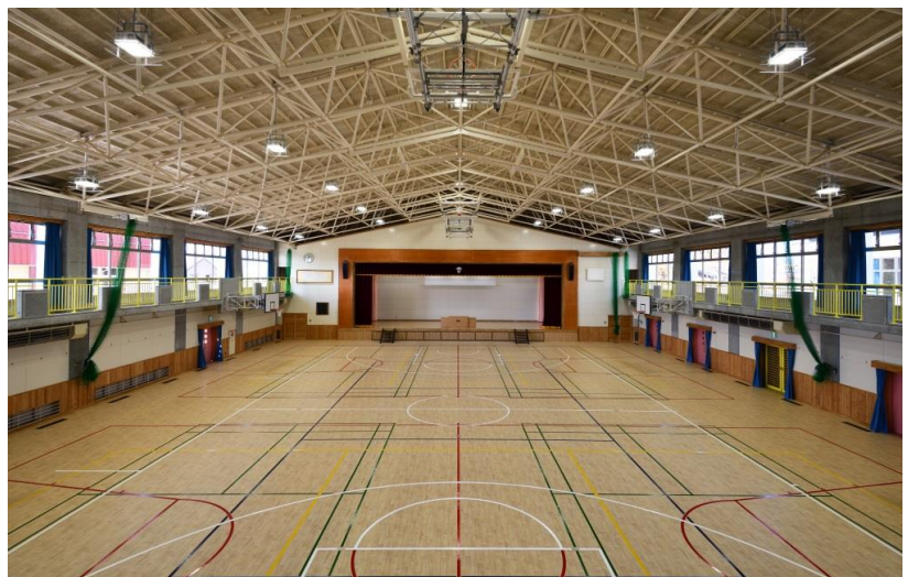
屋内運動場 平家建 1,430.36㎡
