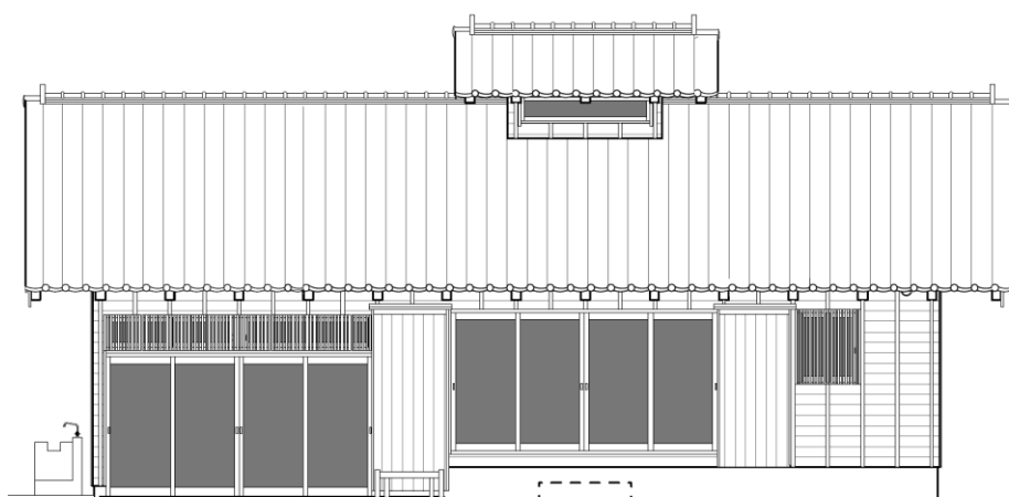
南側立面図
