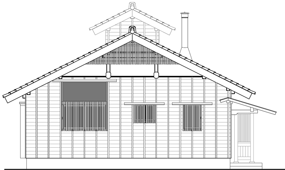
東側立面図
