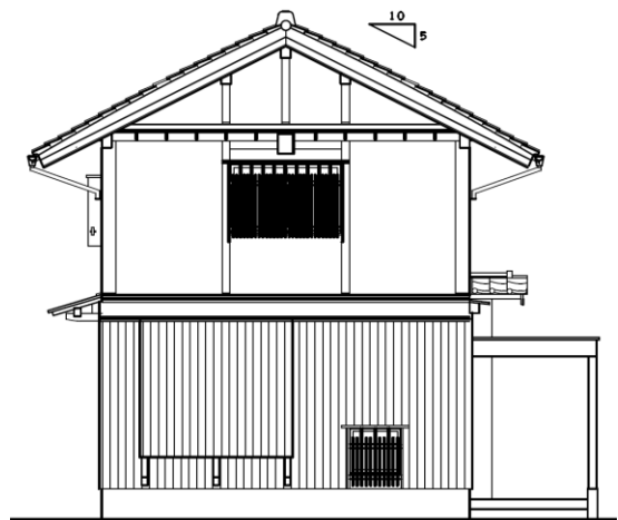
東側立面図
