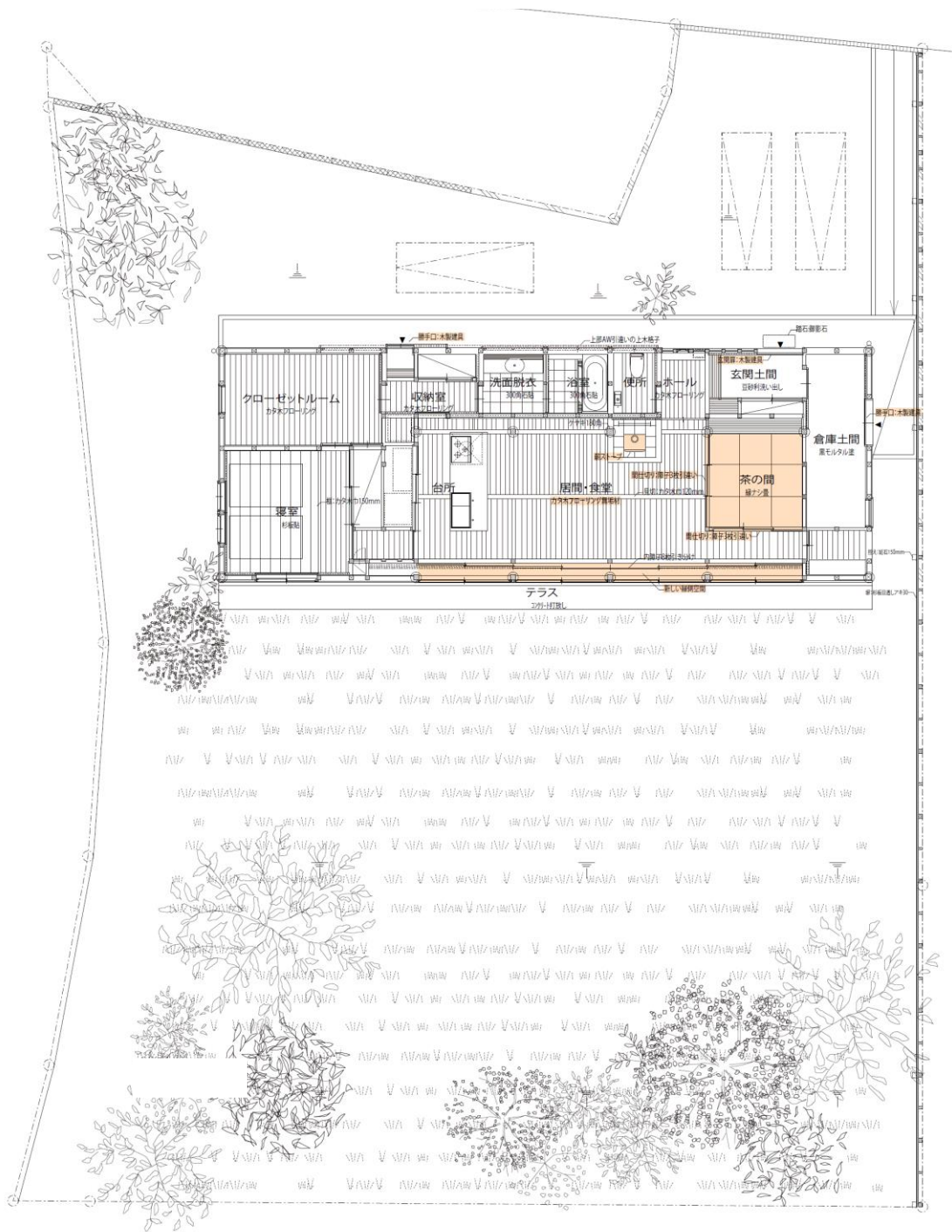
平面図
