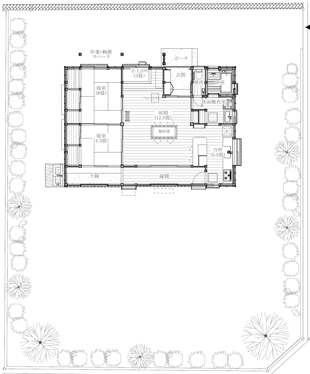
平面図
