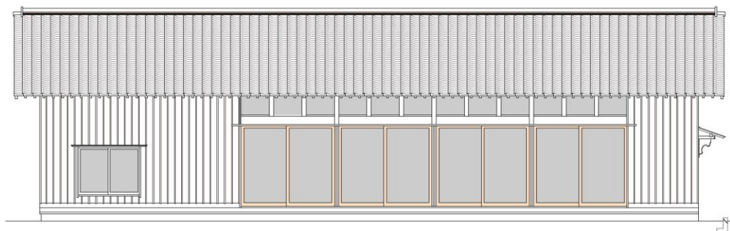
南側立面図
