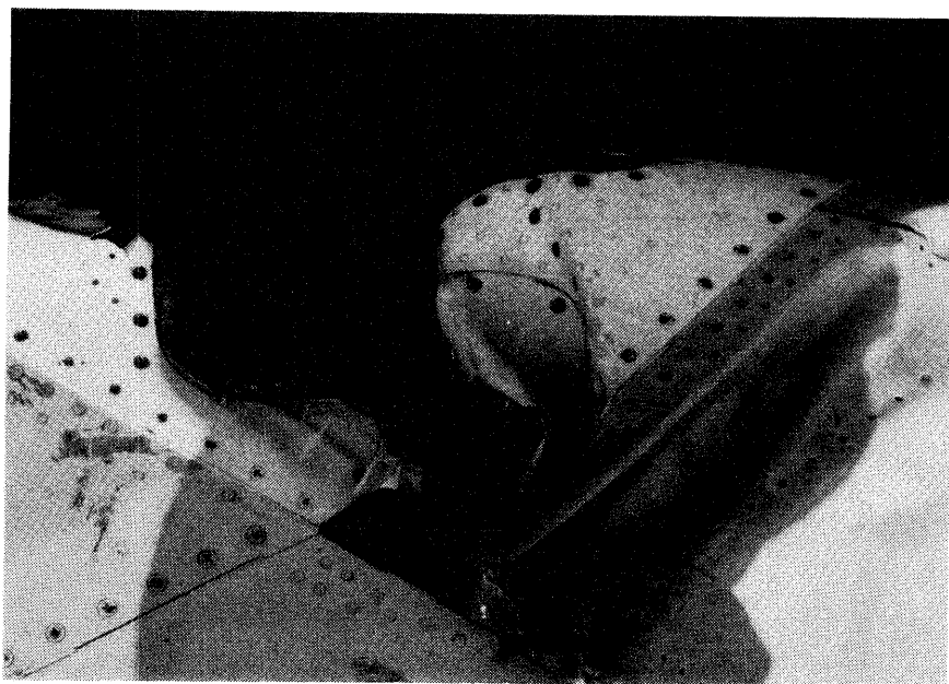
写真 6 右主翼翼端部の損壊状況
