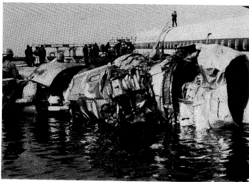
写真16 第1エンジン
