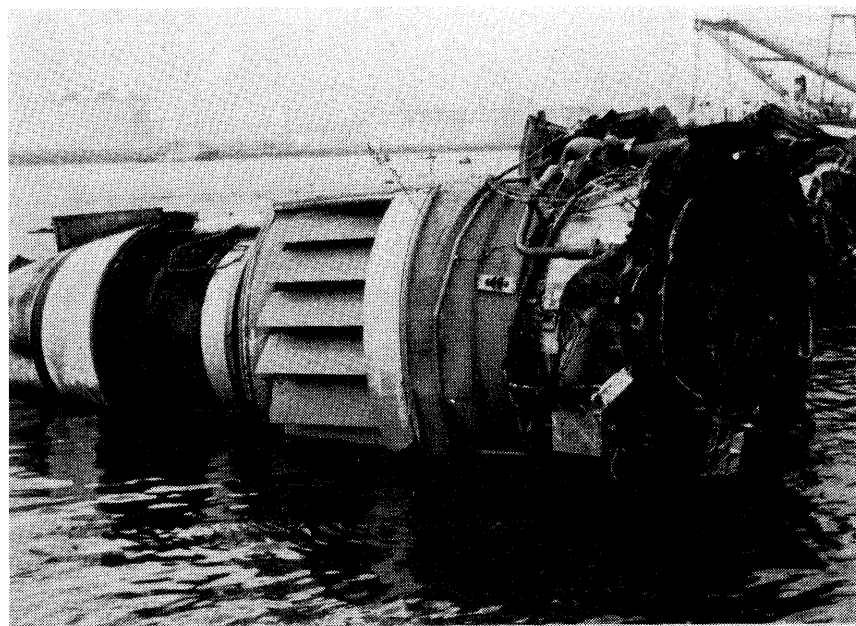
写真 1 9 第 4 エンジン
