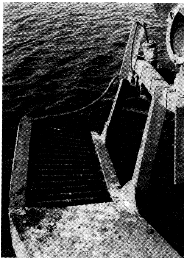
写真 1 3 第 1 5 番進入灯損壊状況（架台）
