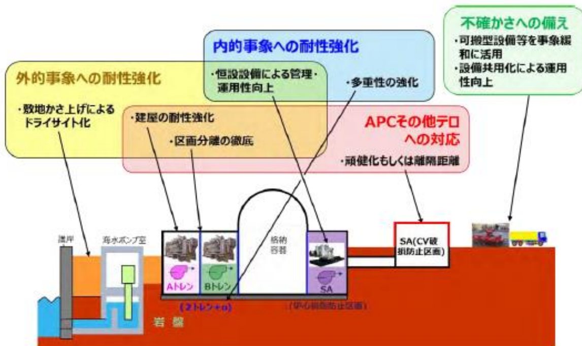
図1 新增設でこそできる合理的でかつ安全性向上を目指す技術要件
