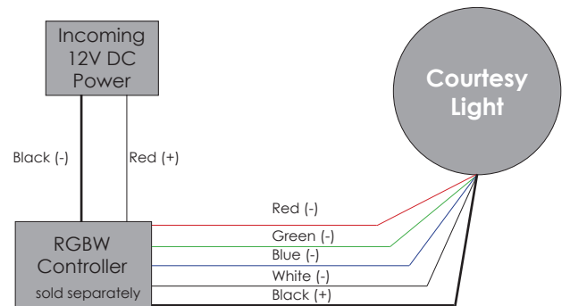
RGBW Wiring
