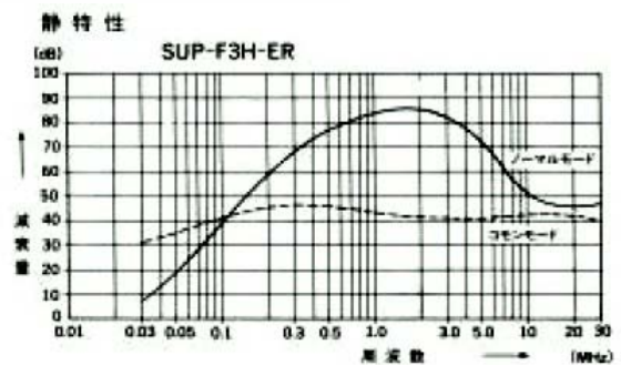
SUP-FHの特性
