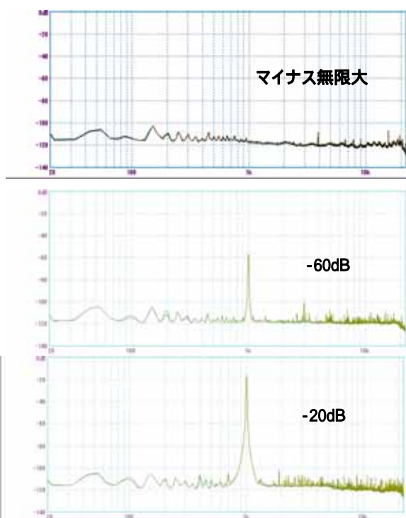
CDプレーヤーのディスプレイ オンとオフとの差 再生CD信号 - 無限大、-60dB、-20dB (差はまったくない)
