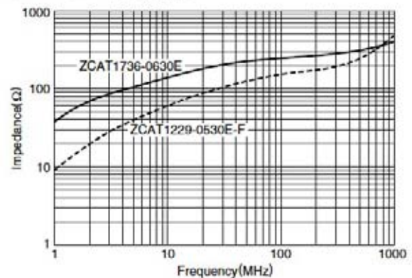
TDK製 ZCAT型インピーダンス特性
