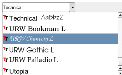
QFontComboBox
