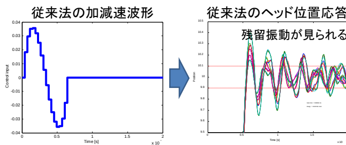
図1. ハードディスク装置のシーク制御 (従来法)
