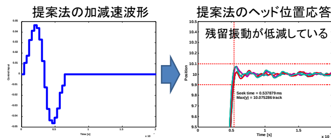
図2. ハードディスク装置のシーク制御 (提案法: 周波数整形終端状態制御)
