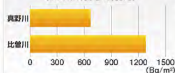
流域面積あたりのセシウム137の流出量 (2013年6月から12月まで)
