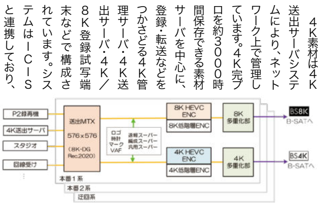
SHV-TOC本線系統概略図
