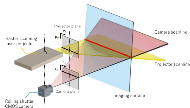
図 1: 本研究で用いるプロジェクターカメラシステムの模式図。
