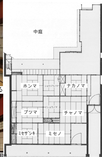
主屋 1階平面図※
