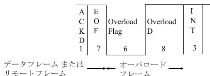
図 3.2c.1-9 オーバロードフレーム
