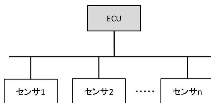
図 3.2c.1-14 SENT の接続構造例
