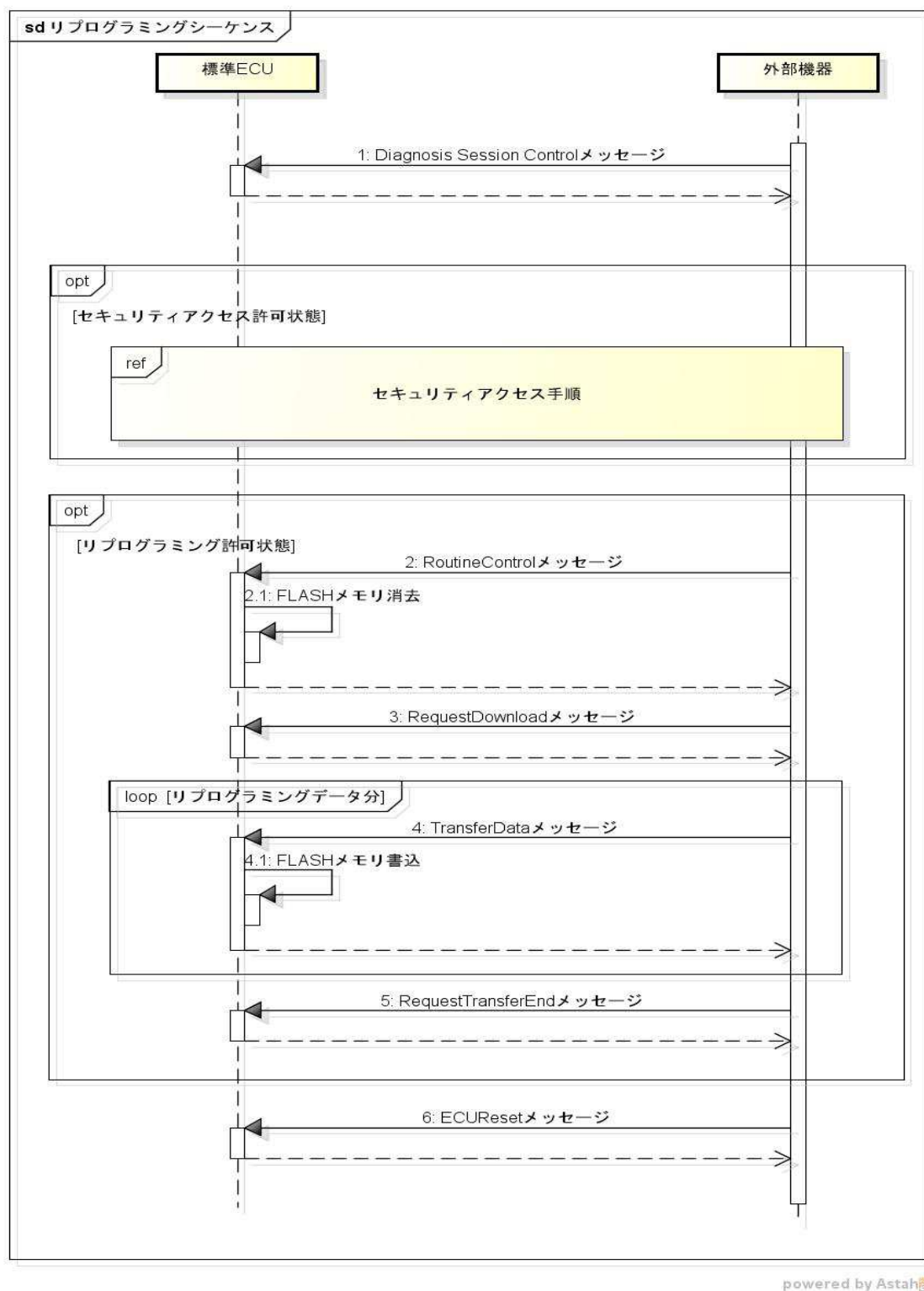
図 3.2a.2-4 リプログラミング手順
