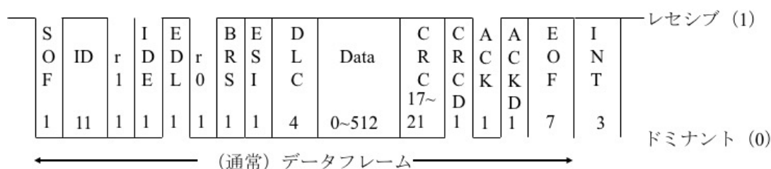
図 3.2c.1-11 CAN-FD データフレーム（標準フォーマット）の各フィールド
