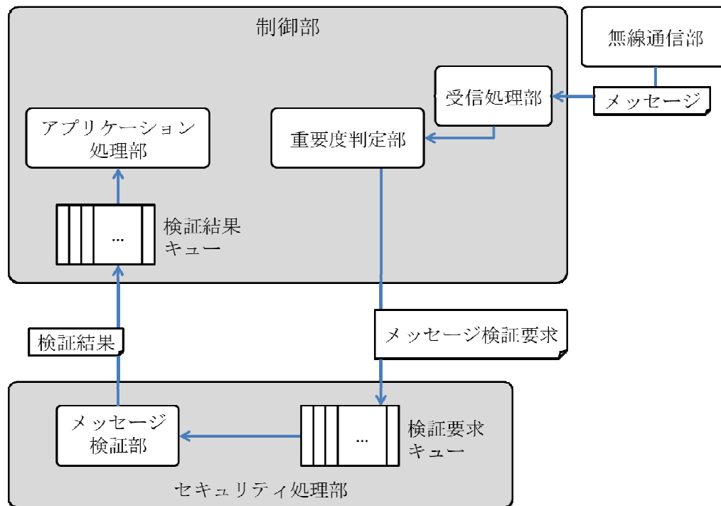
図 3.3.2-3 Verify-on-Demand の処理フロー
