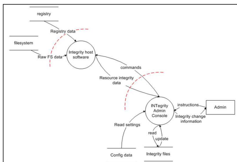
図 3.1.4-6 DFD の例（[28]より引用）
