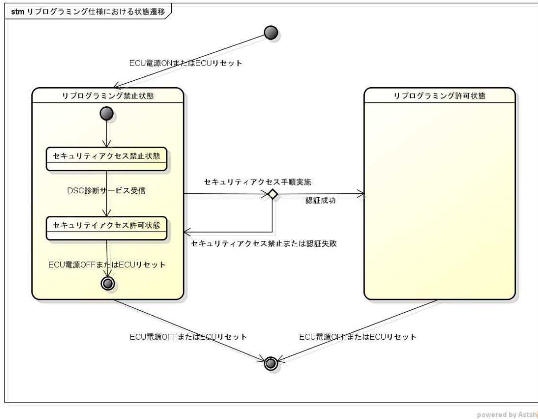
図 3.2a.2-3 リプログラミング仕様における状態遷移
