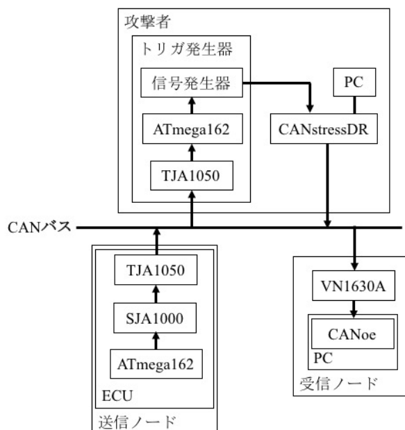
図 3.2c.3-11 CSS 2014 攻撃における実験機器構成
