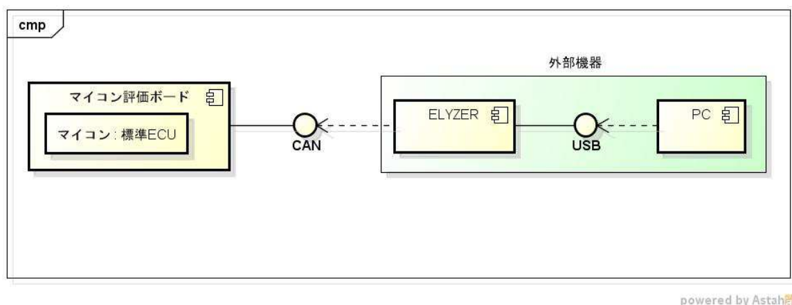
図 3.2a.2-8 リプログラミング評価環境構成
