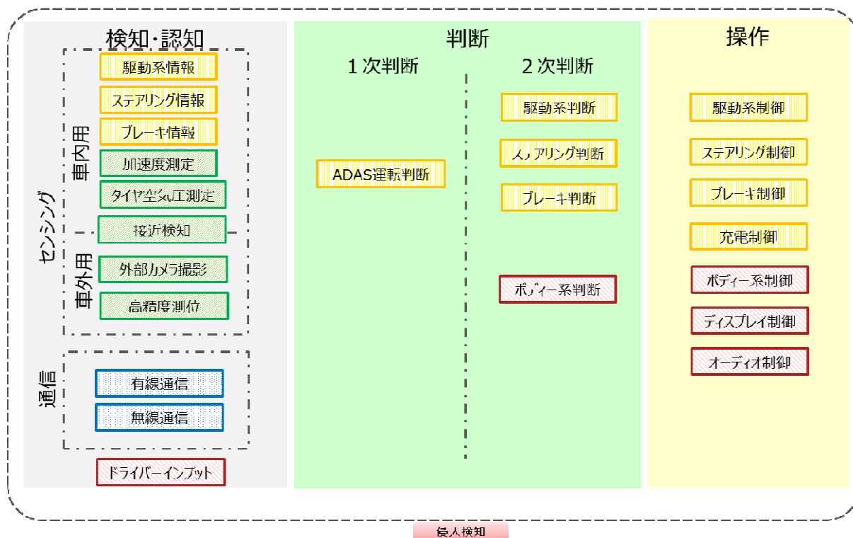
図 3.2b.4-11 全ての CAN バスへの対策概要
