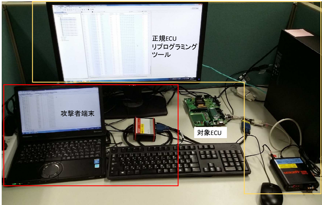
図 3.2d.3-2 攻撃環境の全体図
