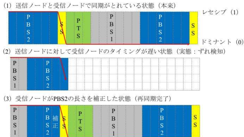
図 3.2c.3-8 受信ノードの再同期手順：受信ノードのエッジが TSEG2 にある場合 （赤実線：CAN バスに流れた電気信号を表す）
