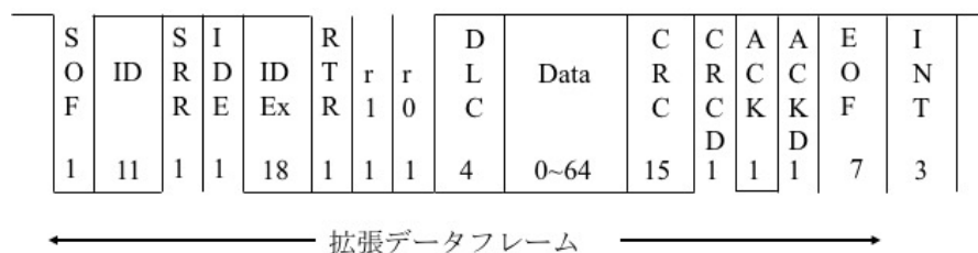
図 3.2c.1-7 拡張データフレーム
