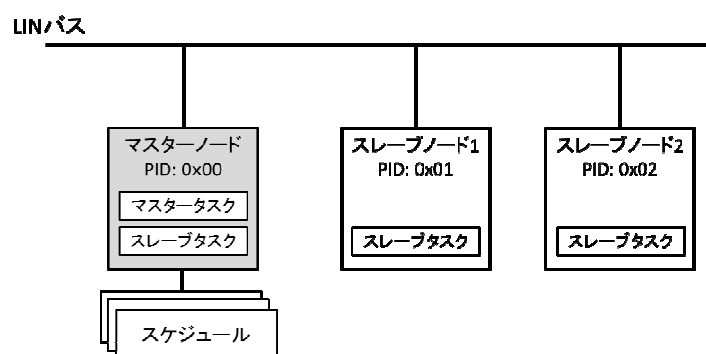
図 3.2c.1-24 LIN の構造
