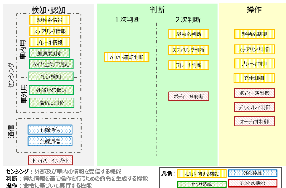
図 3.2b.2-4 自動走行の機能モデル図
