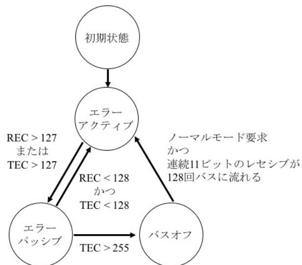
図 3.2c.1-5 エラーカウンタによるノードの状態遷移
