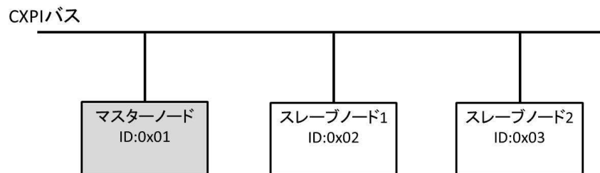
図 3.2c.1-28 CXPI の構造例
