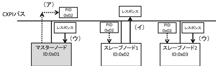
図 3.2c.1-29 イベントトリガ方式の通信手順の例
