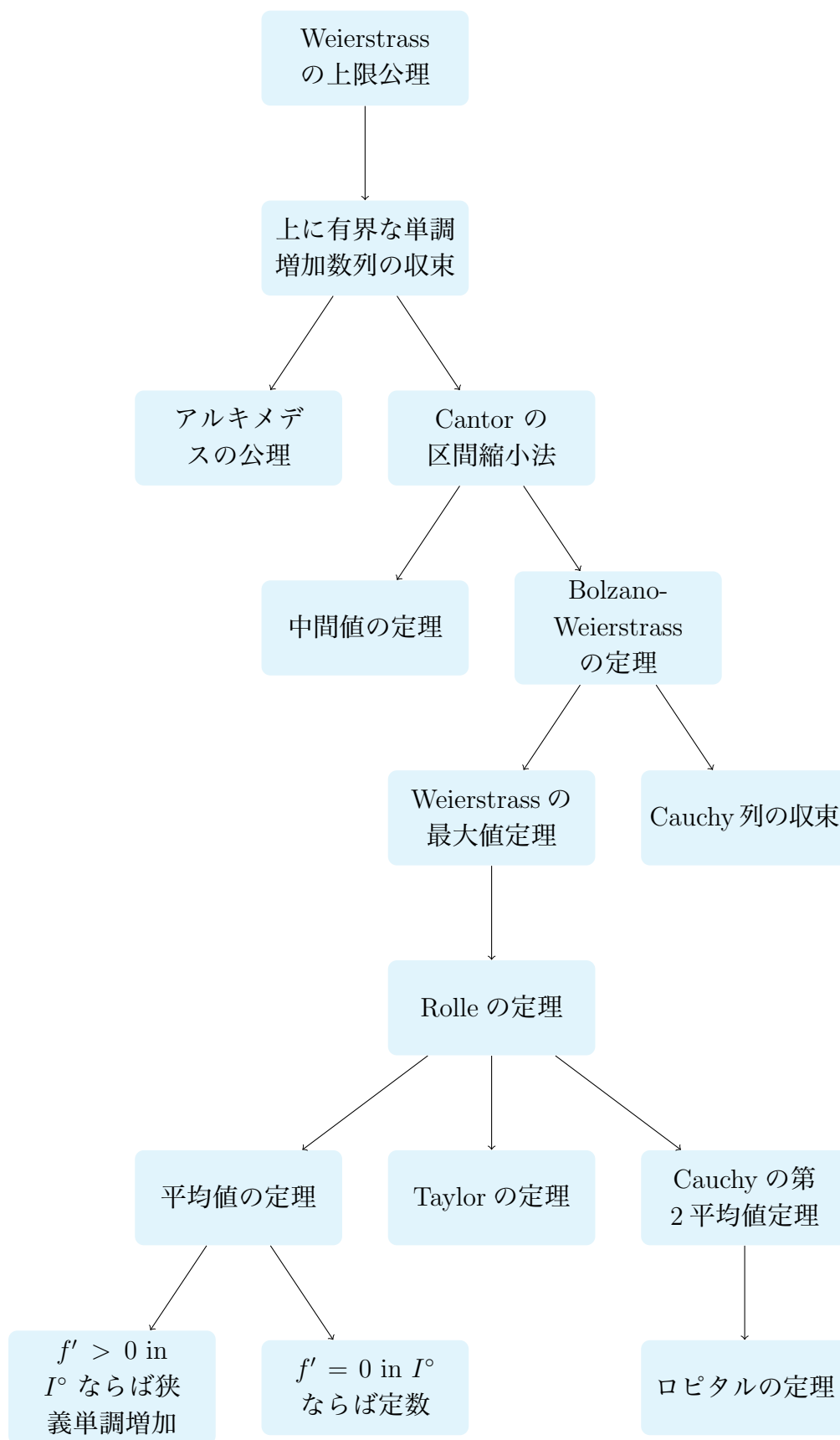
図 1: この講義前半の主要な定理の間の関係
