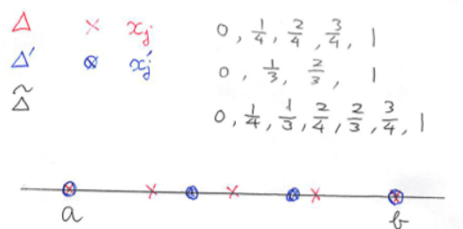
図 5: 2つの分割の分点を合わせて共通の細分を作る
