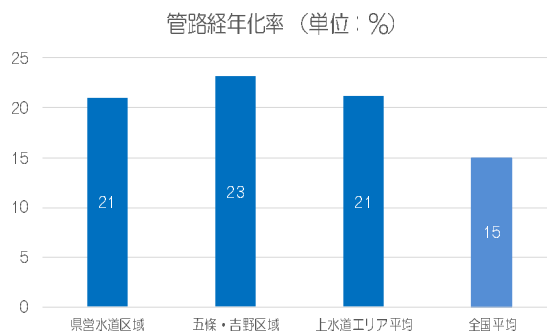
管路経年化率
