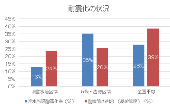
浄水施設・基幹管路の耐震化率
